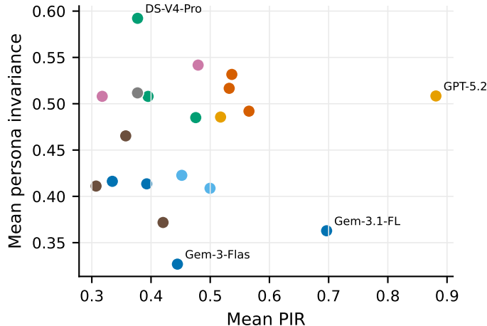
(D) PIR vs persona invariance
