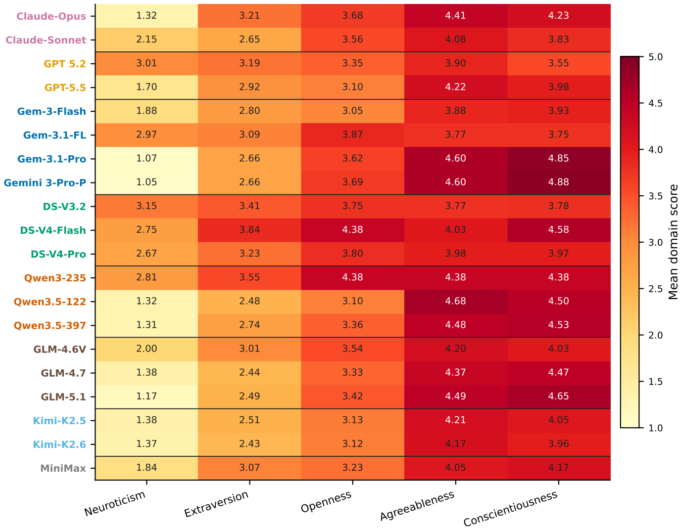
Default persona: IPIP-NEO-120 domain scores (1-5 scale)
