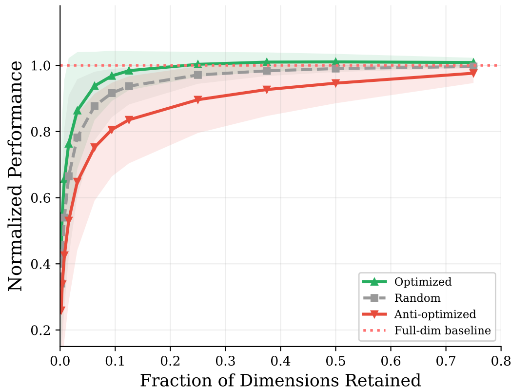
Stella EN 400M (1024d)
