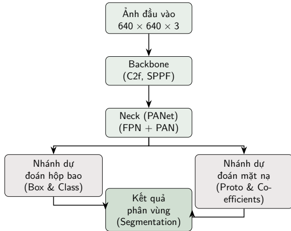
Hình 5: Sơ đồ kiến trúc YOLO26-seg
