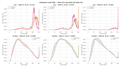
Hình 4: Histogram RGB của các cặp bệnh dễ nhầm lẫn
