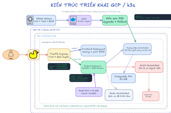
Hình 8: Kiến trúc tổng thể hệ thống trên GCP và k3s
