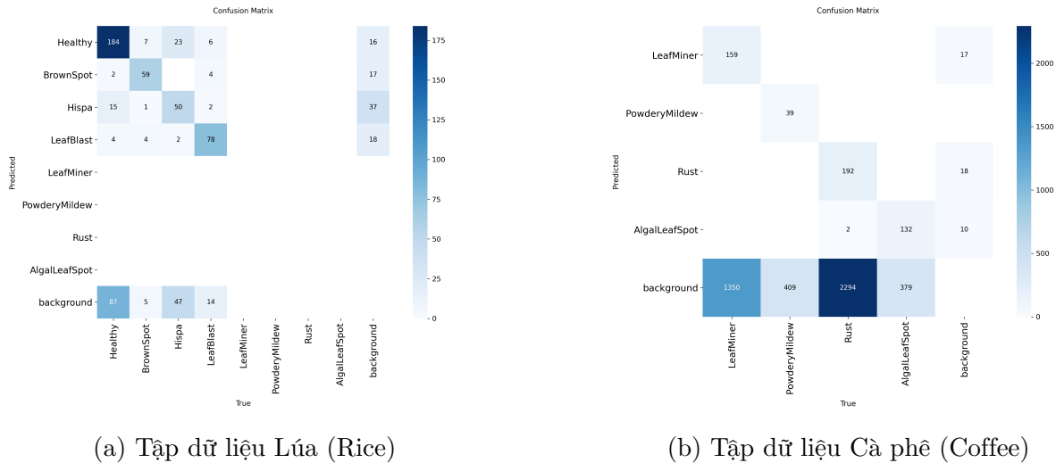
Hình 12: Ma trận nhầm lẫn (Confusion Matrix) của mô hình YOLO26-seg
