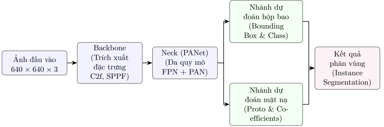
Hình 10: Sơ đồ kiến trúc chi tiết của mô hình YOLO26-seg dùng cho phân vùng vết bệnh
