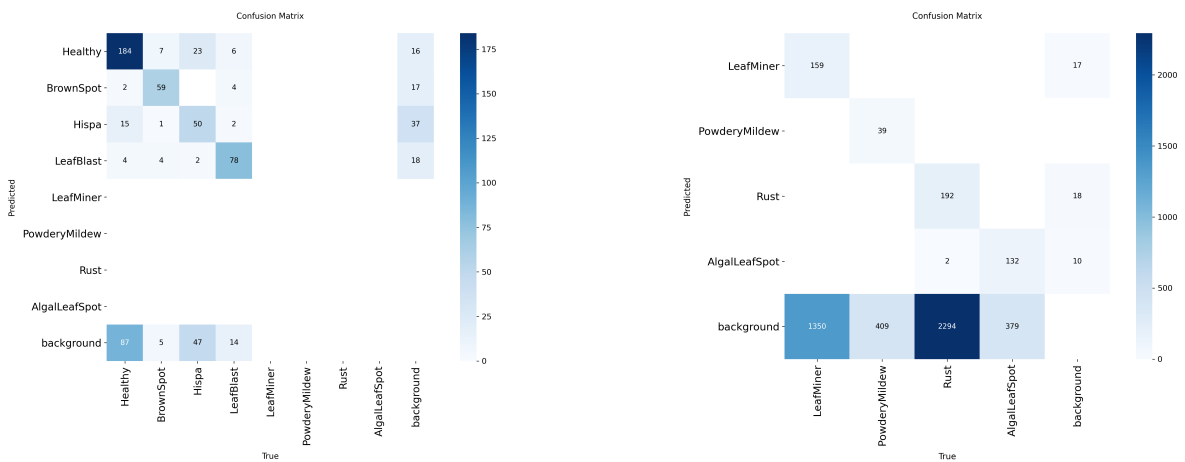
Hình 12: Ma trận nhầm lẫn (Confusion Matrix) của mô hình YOLO26-seg
