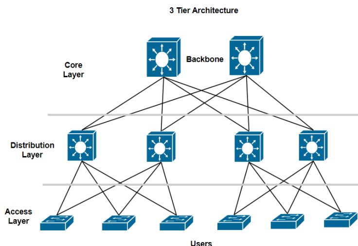
Hình 2.1 Mô hình mạng Campus Core–Distribution–Access
