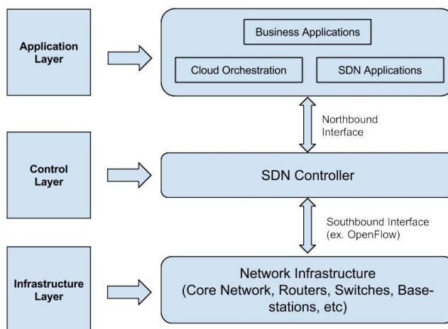
Hình 2.3 Kiến trúc ba lớp của SDN
