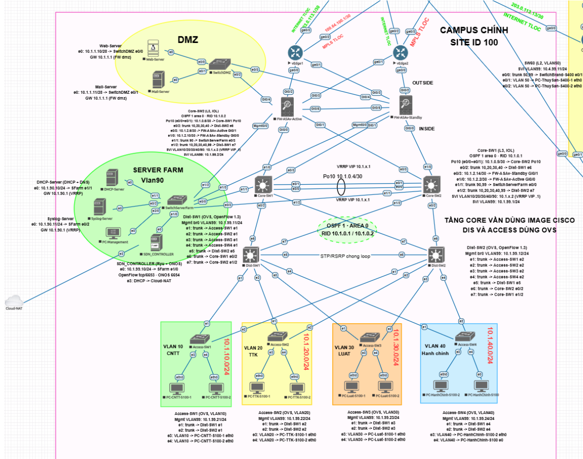
Hình 3.3 Sơ đồ chi tiết Campus chính (Site 100) trên EVE-NG
