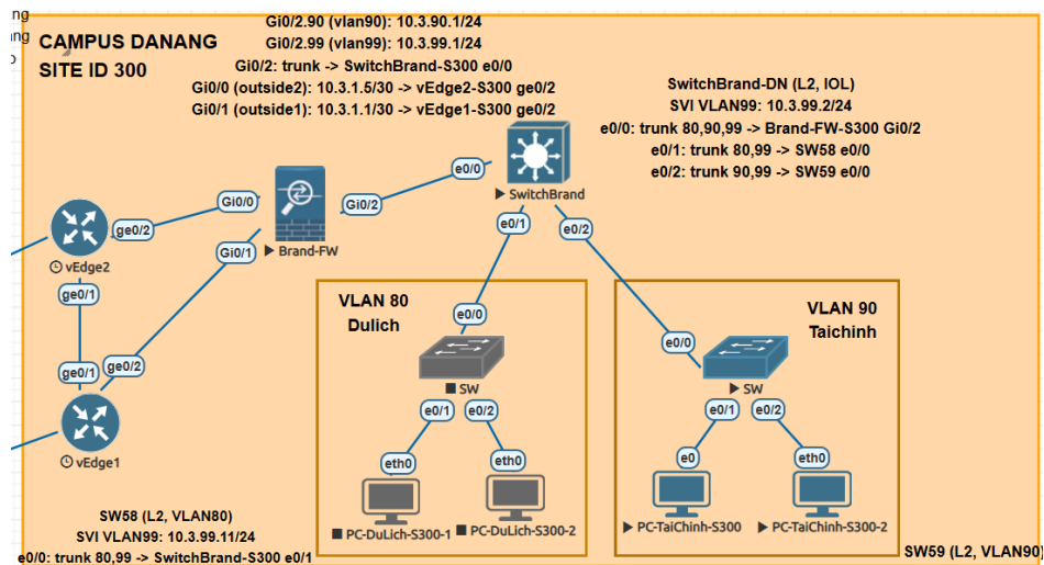
Hình 3.5 Sơ đồ chi nhánh Đà Nẵng (Site 300)
