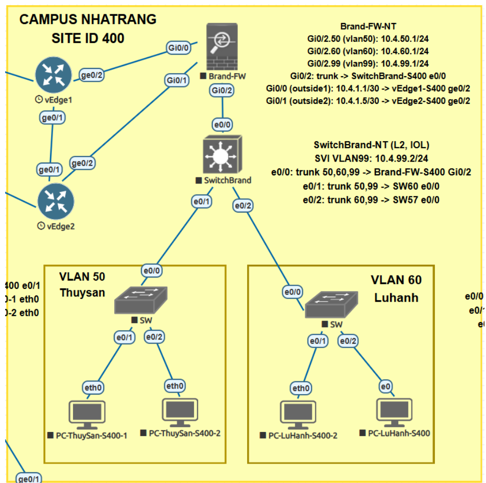
Hình 3.6 Sơ đồ chi nhánh Nha Trang (Site 400)
