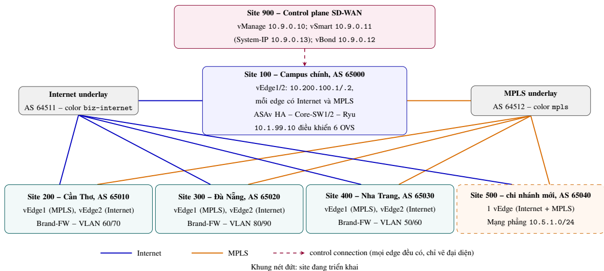
Hình 3.1 Topology logic của hệ thống tại thời điểm giữa kỳ
