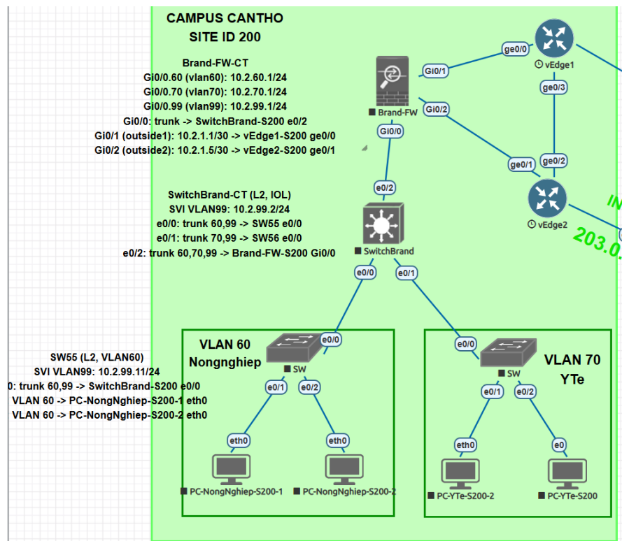
Hình 3.4 Sơ đồ chi nhánh Cần Thơ (Site 200)
