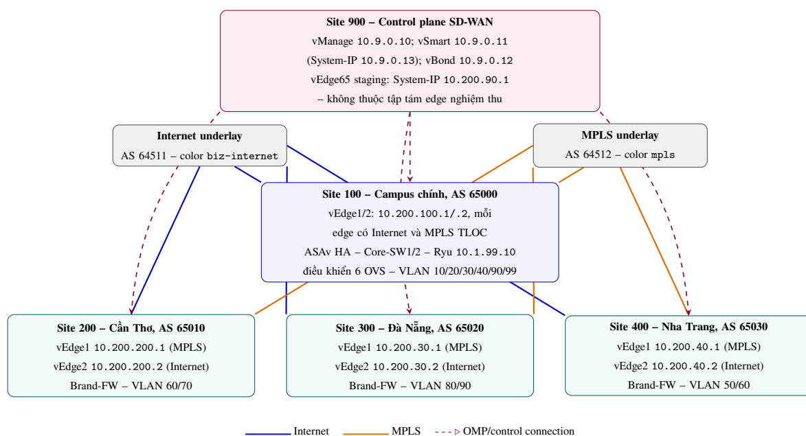
Hình 3.2 Topology logic đã chuẩn hóa theo cấu hình hiện hành
