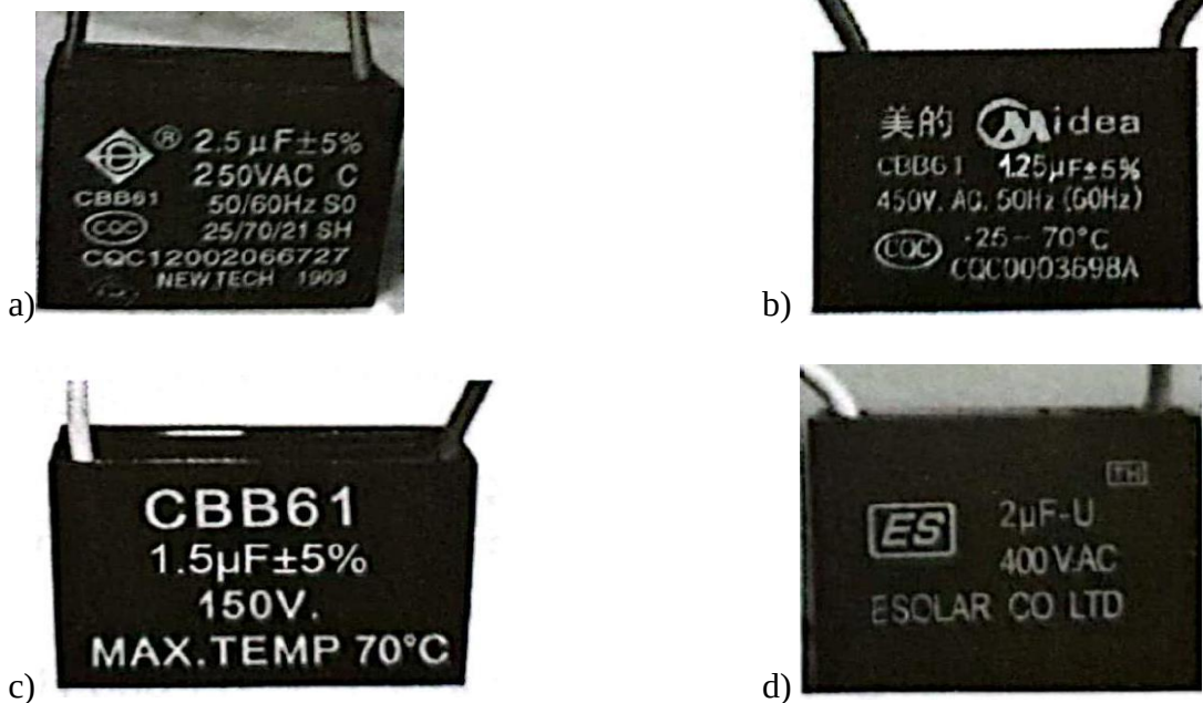
Hình 21.6. Một số tụ điện dùng cho quạt điện
