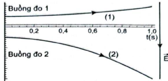
Hình 18.3. Quỹ đạo chuyển động của hai hạt trong một giây sau tán xạ ở hai buồng đo với cùng tỉ lệ kích thước
