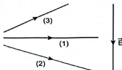
Hình 18.2. Quỹ đạo chuyển động của ba hạt sinh ra sau tán xạ đi trong điện trường đều \vec{E}
