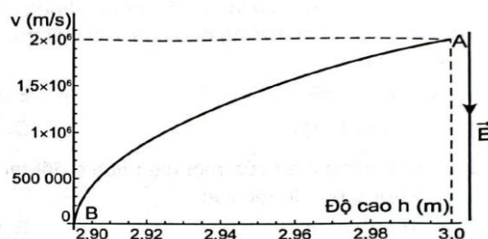
Hình 19.1. Đồ thị tốc độ thay đổi theo độ cao của một electron chuyển động trong điện trường của Trái Đất
