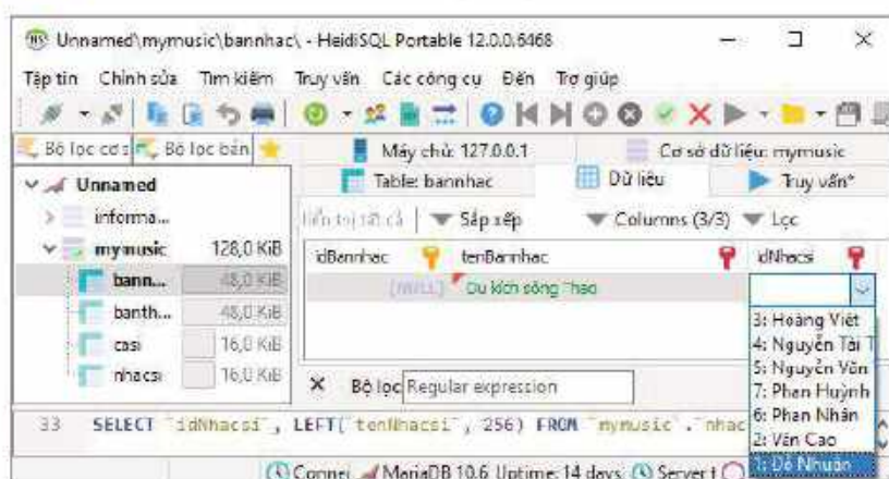
Hình 22.3. Nhập dữ liệu cho trường khoá ngoài
