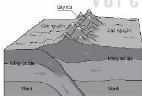
Mảng lục địa và mảng lục địa
