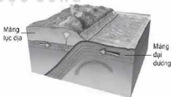
Mảng lục địa và mảng đại dương
