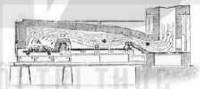
Hình 6. Lò luyện quặng theo phương pháp "puť-ding"
