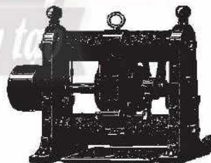
Hình 11.3. Máy phát điện một chiều của G. Đi-na-mô
