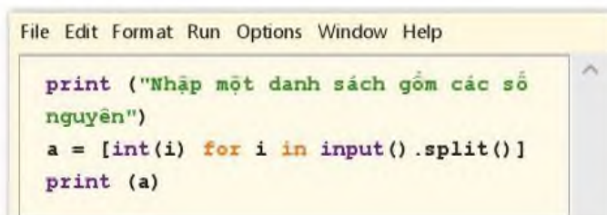
Hình 2a. Một chương trình nhập danh sách các số nguyên và in ra danh sách đó
