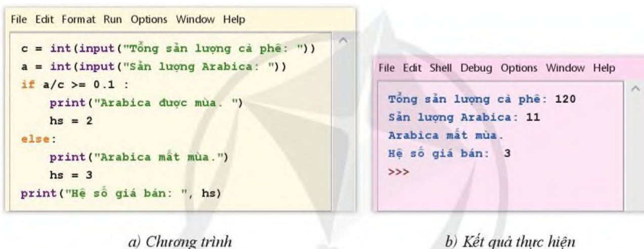
Hình 7. Chương trình đánh giá sản lượng cà phê ở Tây Nguyên
