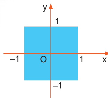
Hình 5.2. Hình vuông trong mặt phẳng tọa độ
