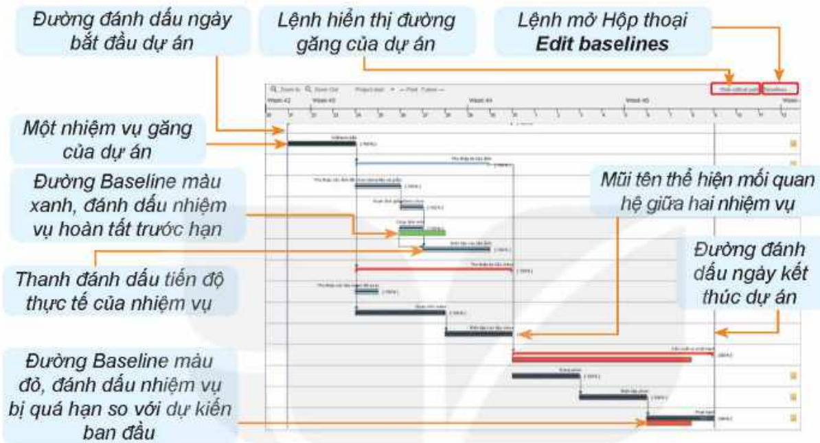
Hình 4.1. Biểu đồ Gantt của một dự án
