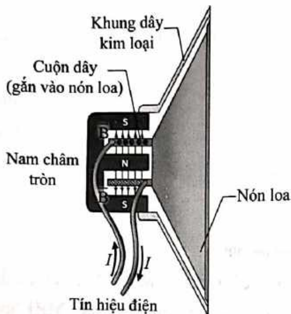
a) Cấu tạo đơn giản của loa
