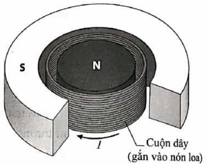
b) Bố trí của cuộn dây và nam châm bên trong loa
