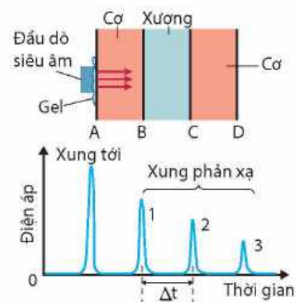
Hình 7.5. Các xung siêu âm trong siêu âm kiểu A
