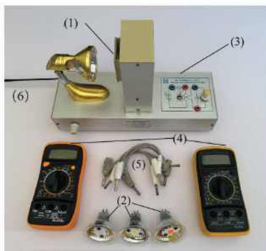
Hình 9.6. Bộ thiết bị khảo sát dòng quang điện
