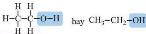
Hình 26.2 Công thức cấu tạo của ethyl alcohol
