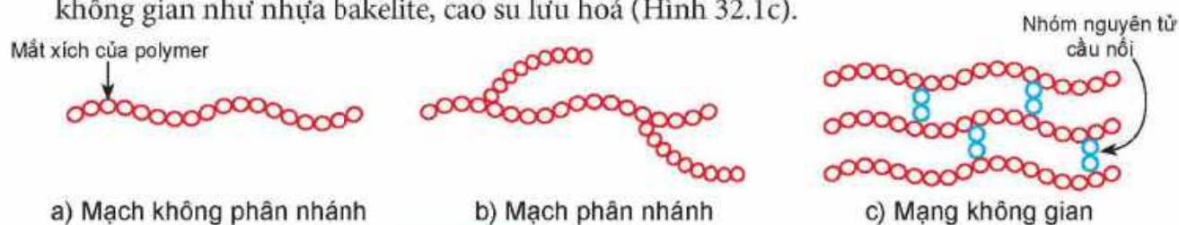
Hình 32.1 Các loại mạch polymer
