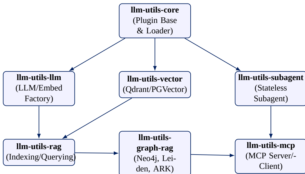
Hình 4.1: Sơ đồ Phụ thuộc Mô-đun trong uv Workspace Monorepo
