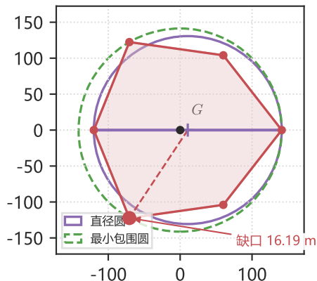
(b) 算例 G: \pm 1^\circ 放大为 \pm 8^\circ , 直径圆盖不住 P
