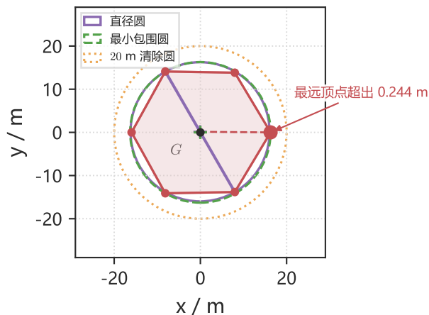
(c) 算例 G 真实 \pm 1^\circ : R_{MEC} = 16.288 < 20 m, 可清除
