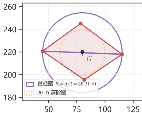
(d) 算例 B: 覆盖, R_{MEC} = 35.209 > 20 m, 不可清除
