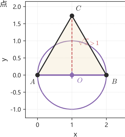
(b) 反例：第三顶点在直径圆外
