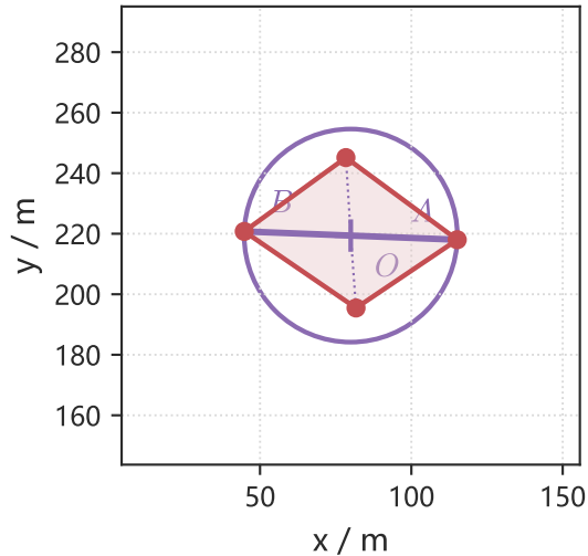
(a) 圆心取直径中点，再量各顶点到中点
