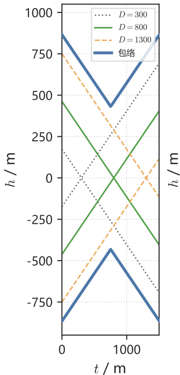
(b) 对顶锥族与包络
