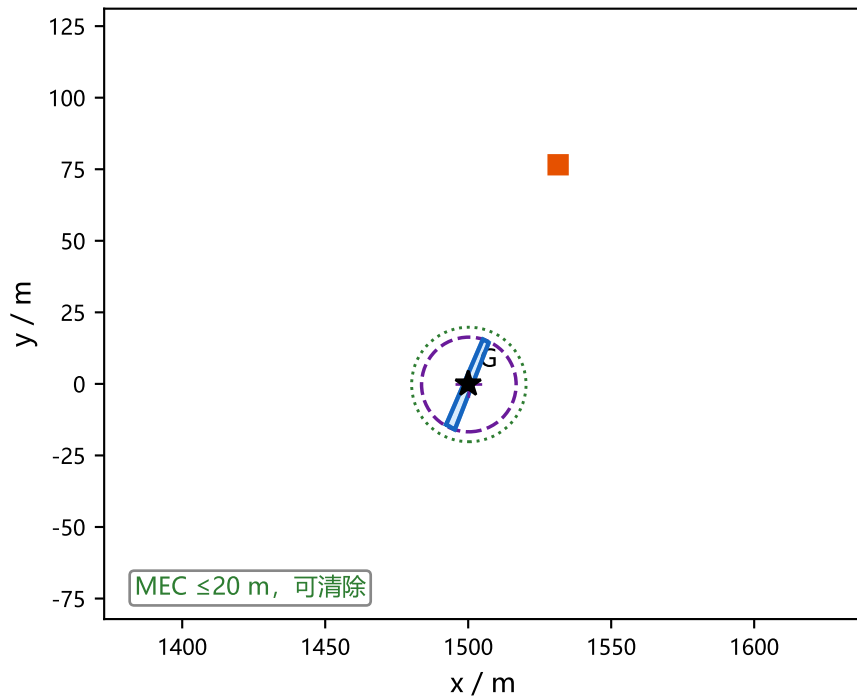
(b) 长轴切割后再测 直径 33.1 \text{ m} , MEC 16.5 \text{ m}
