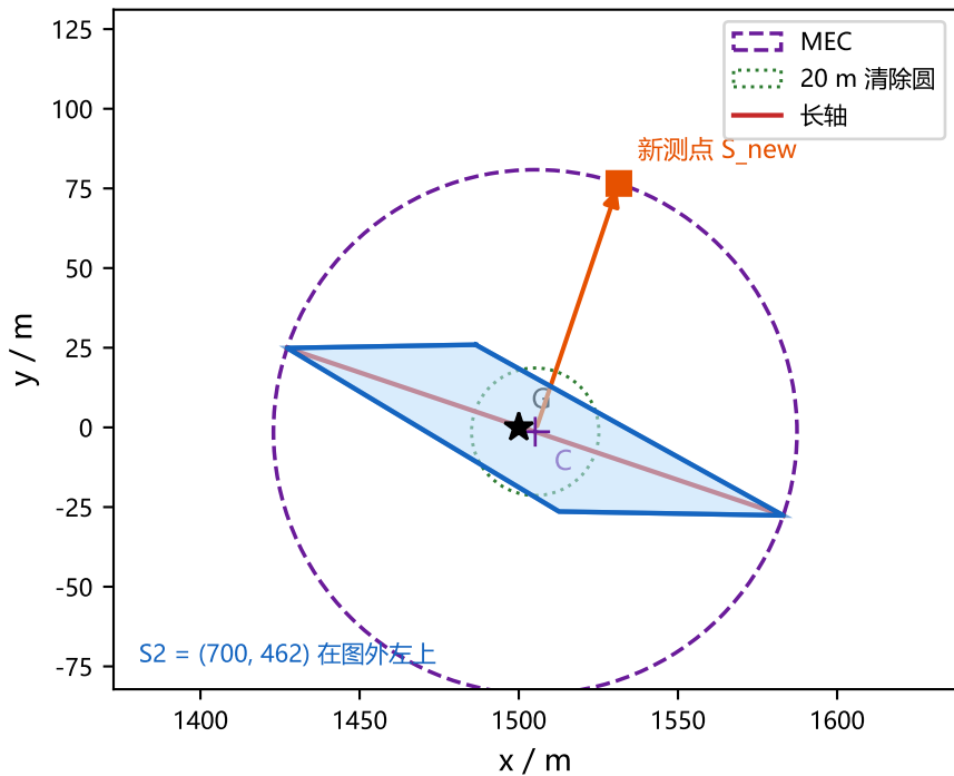
(a) 两次测向后 直径 164.5 \text{ m} , MEC 82.2 \text{ m}
