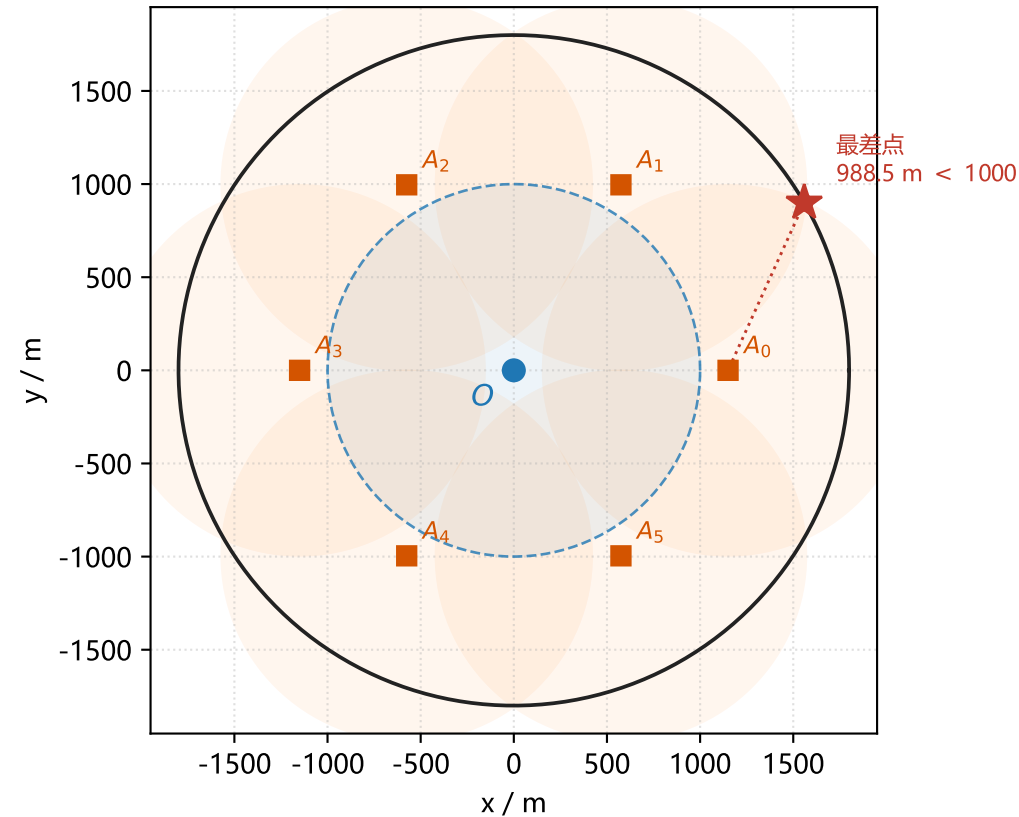
(a) 覆盖网：原点 + 1150 m 六等分点
