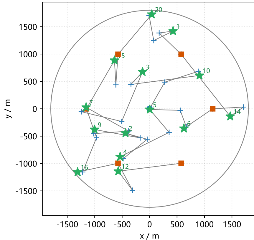
(b) 演练轨迹 (星号为清除点, 数字为频道)
