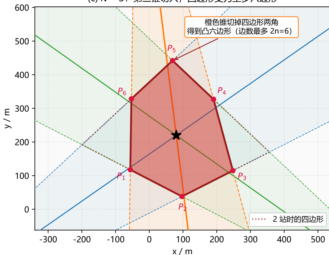
(c) N = 3 : 第三锥切入，四边形变为至多六边形
