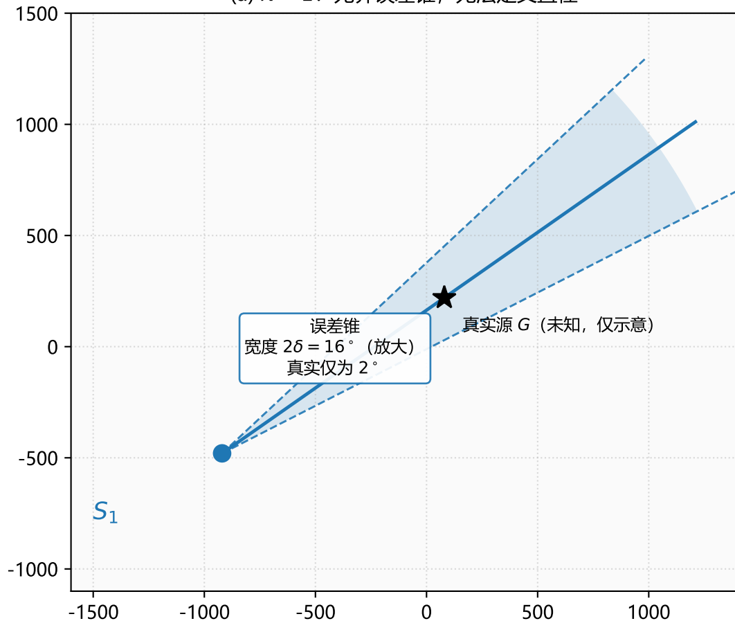
(a) N = 1 : 无界误差锥，无法定义直径
