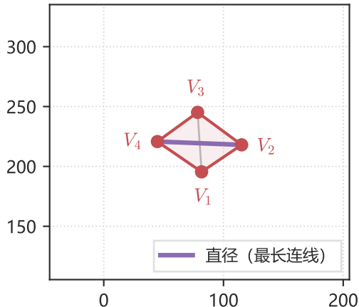
(b) 全部顶点连线, 最长者为直径
