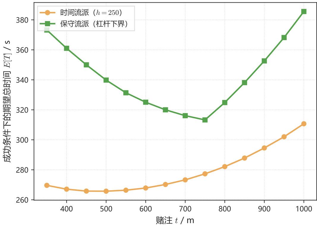
序贯仿真：成功清除的期望时间
