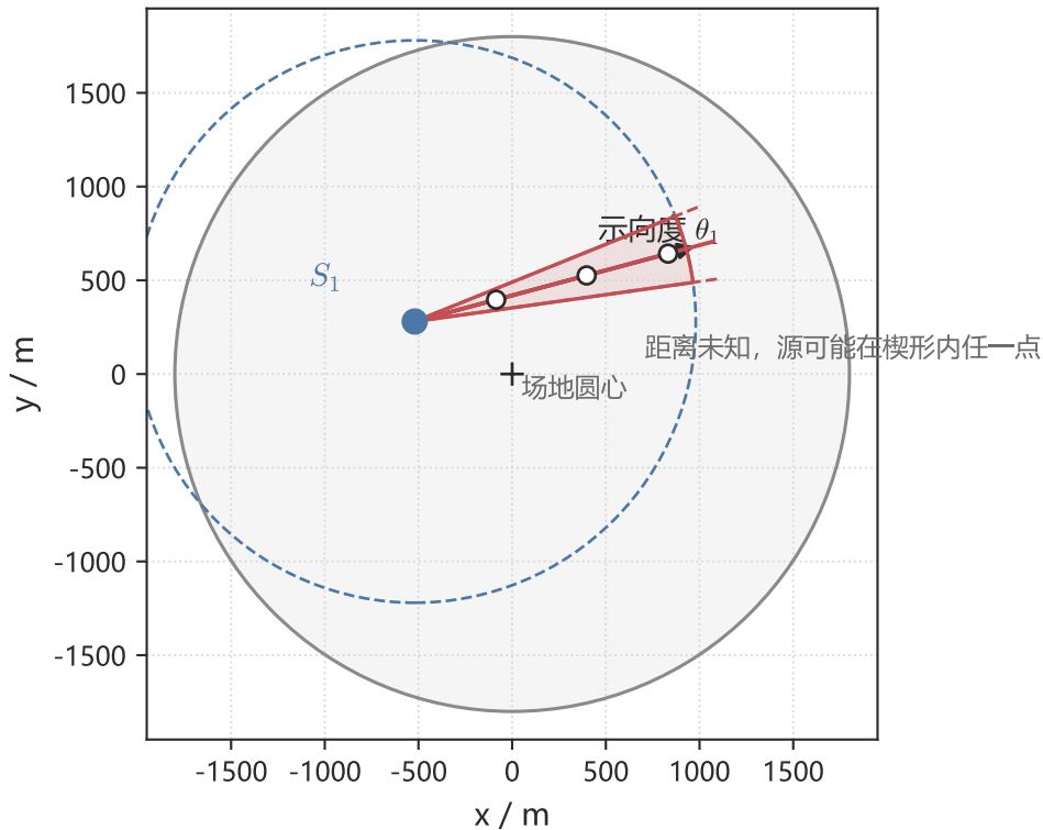
第一次测向后：干扰源落在 S_1 示向度的楔形里
