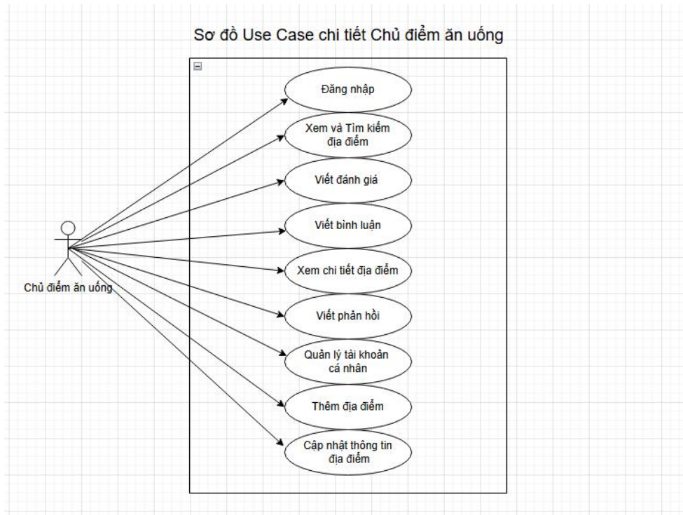
Hình 3.6 Sơ đồ Use Case chi tiết Chủ điểm ăn uống (điểm kinh doanh)
