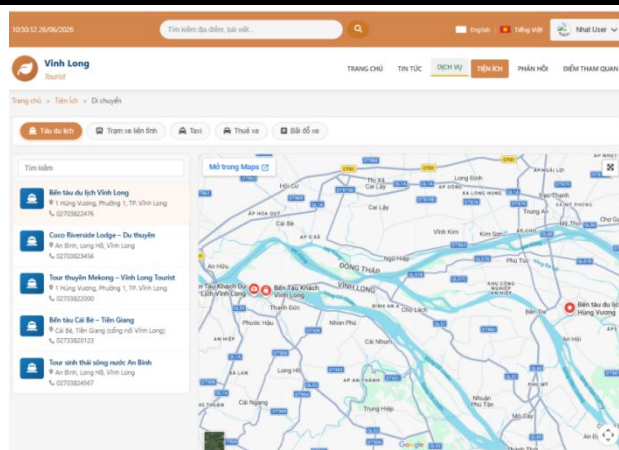
Hình 4.19. Giao diện Chi tiết tiện ích - Các phương tiện di chuyển
