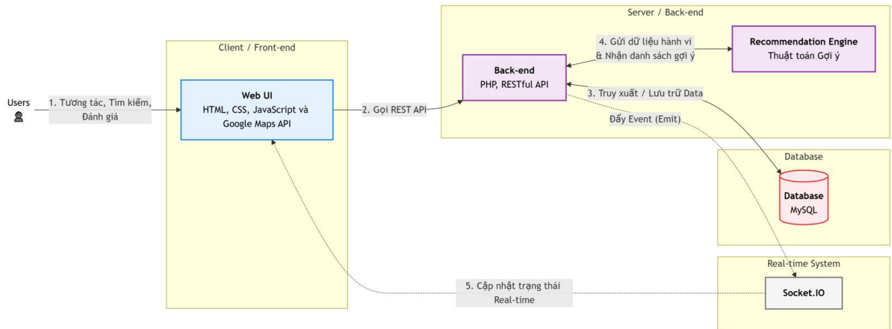
Hình 3.1. Kiến trúc tổng thể hệ thống Vĩnh Long Tourist
