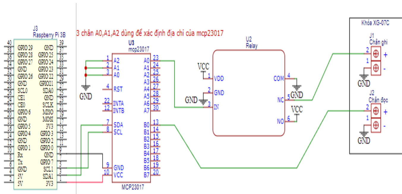
Sơ đồ nguyên lý phần cứng
