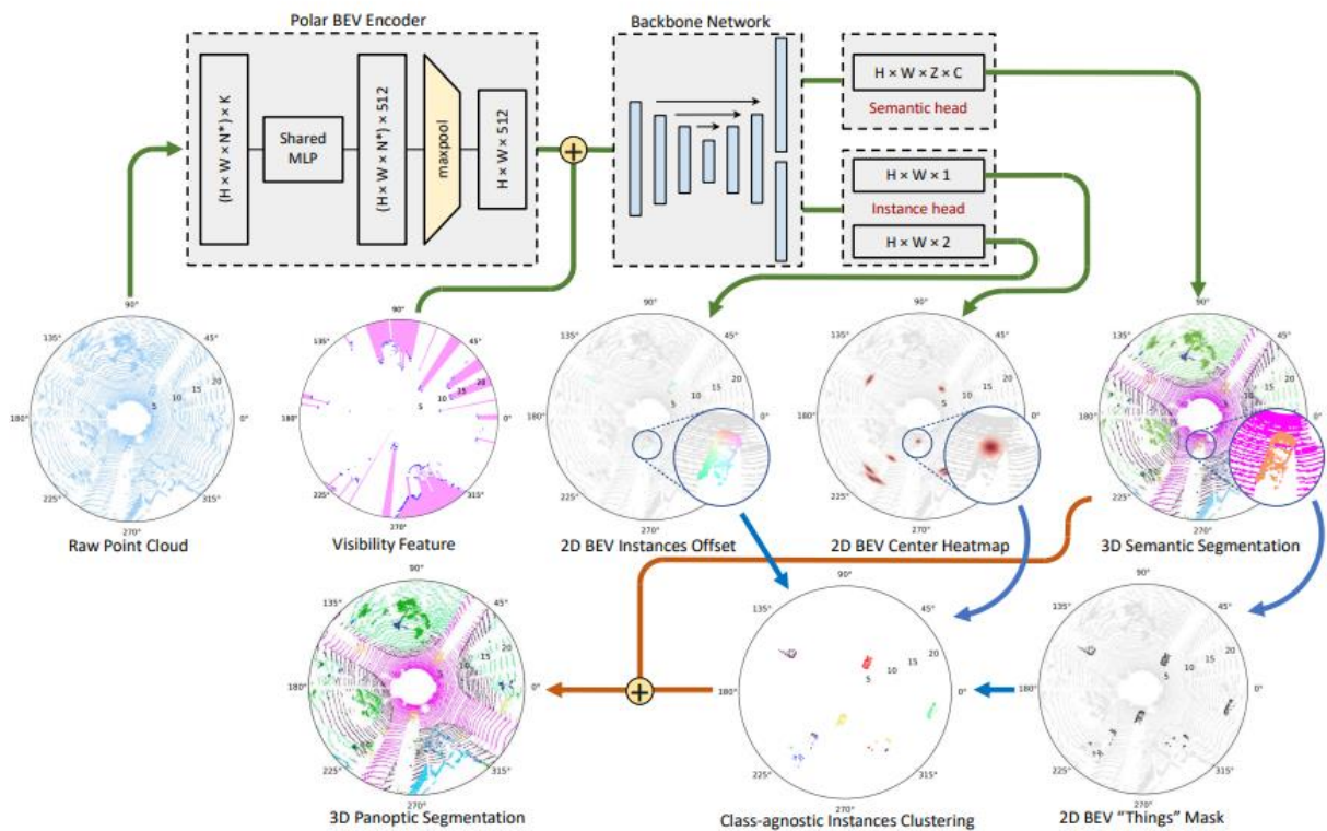
Cấu trúc model
