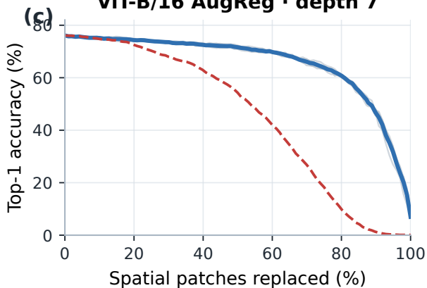
ViT-B/16 AugReg · depth 7
