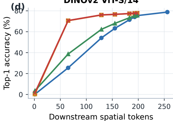
DINOv2 ViT-S/14
