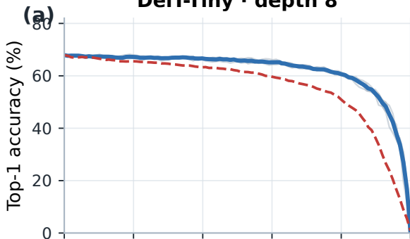
DeiT-Tiny · depth 8
