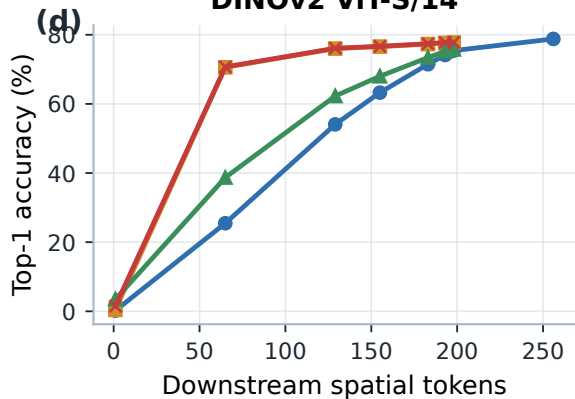
DINOv2 ViT-S/14
