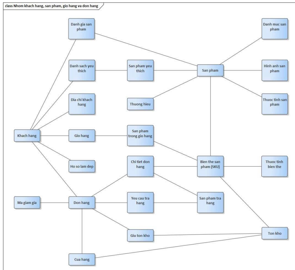
Hình 4.1. Lược đồ logic - nhóm khách hàng, sản phẩm, giỏ hàng và đơn hàng
