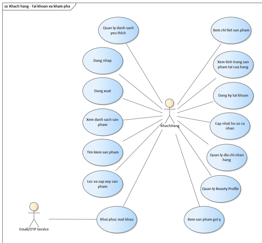
Hình 3.0.2 Khách hàng- Tài khoản và khám phá
