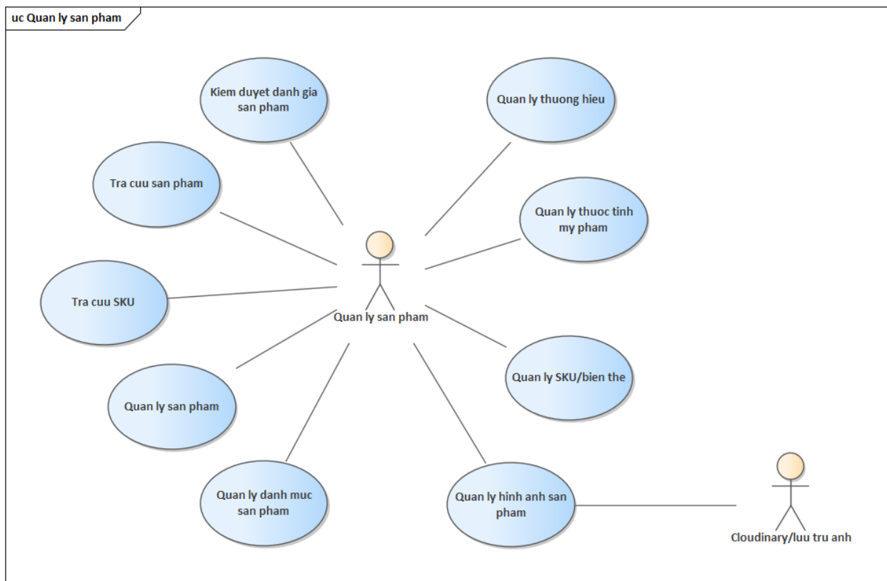
Hình 3.0.4 Quản lý sản phẩm
