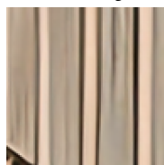
IMDN
