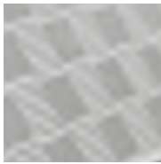
Bicubic
