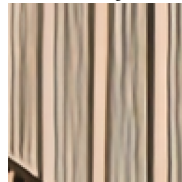
DPRNet (ours)
