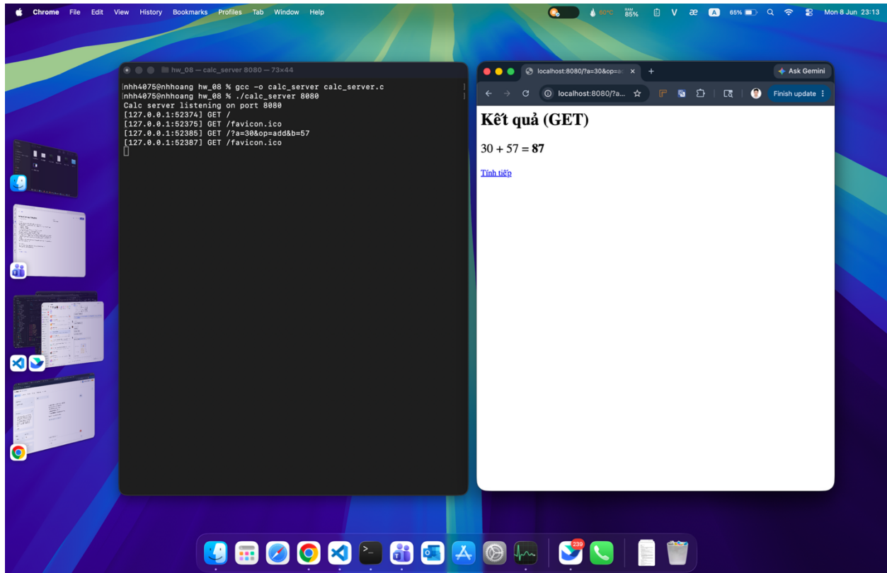
Hình 2: Demo trình duyệt nhận được kết quả phép cộng bằng GET
