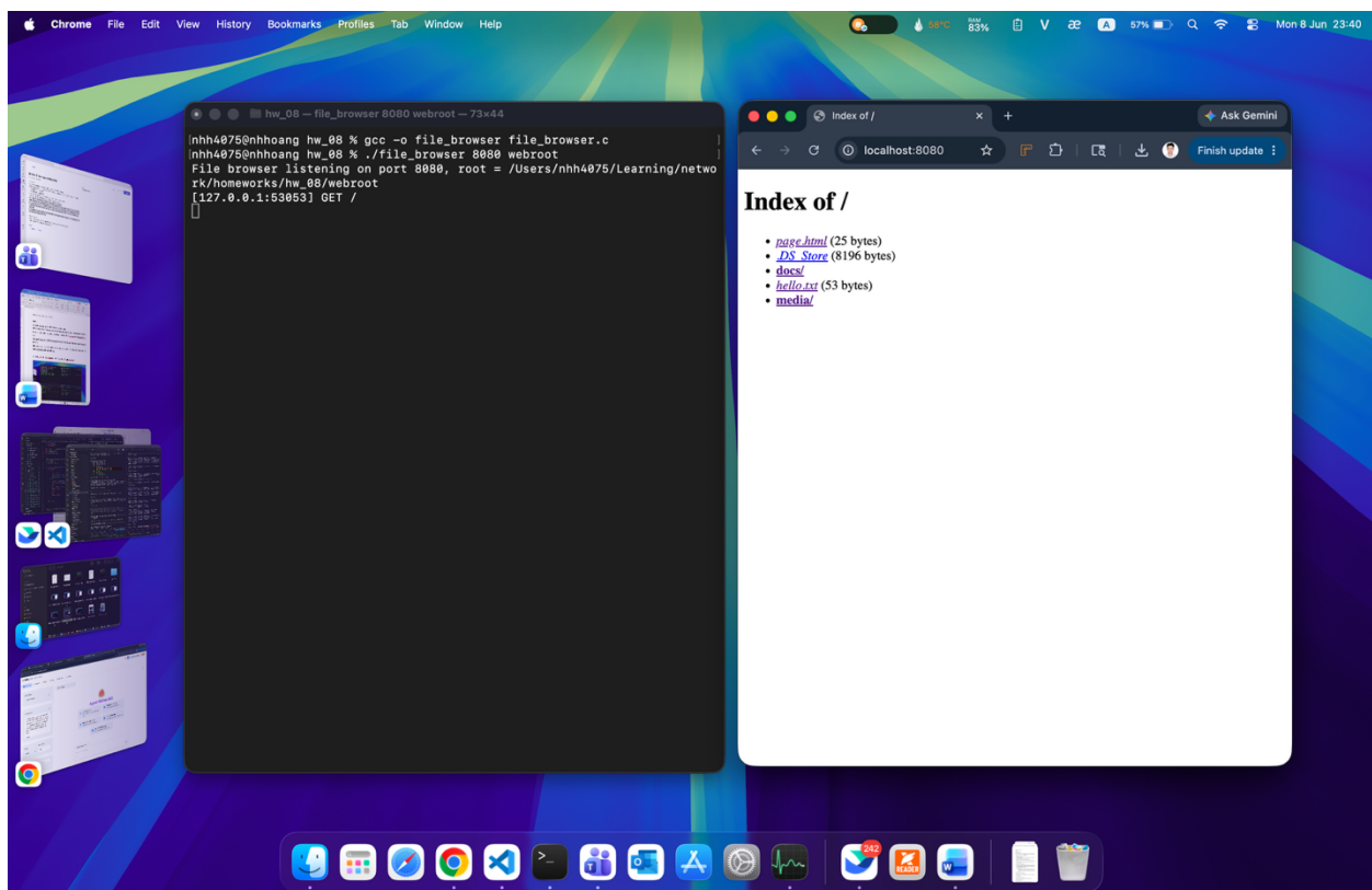
Hình 5: Demo trình duyệt truy cập được đến File HTTP Server ở thư mục gốc
