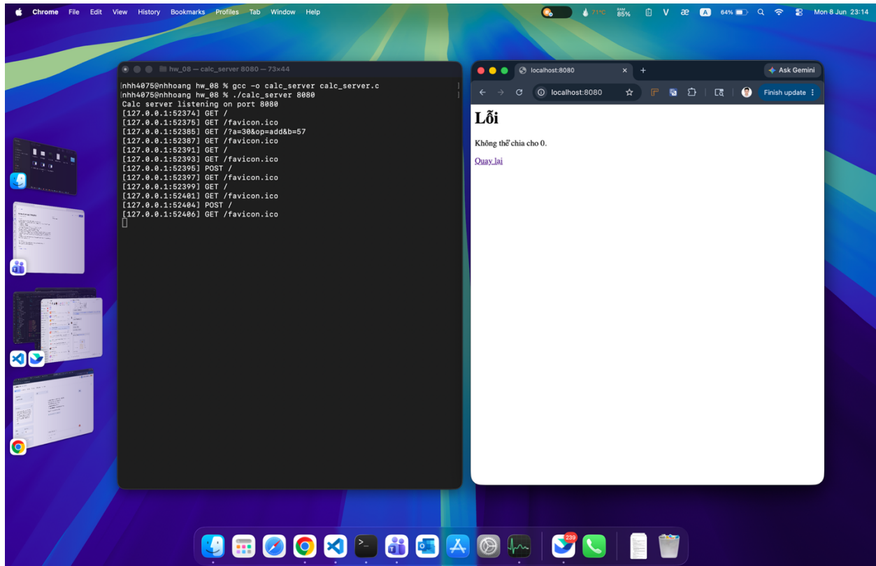
Hình 4: Demo trình duyệt nhận được báo lỗi phép chia cho 0
