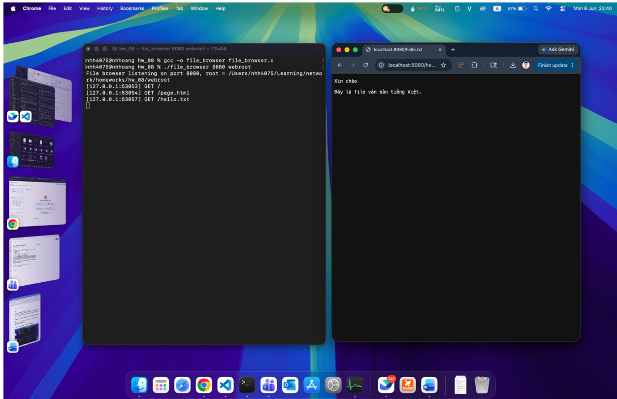
Hình 6: Demo trình duyệt xem được file văn bản
