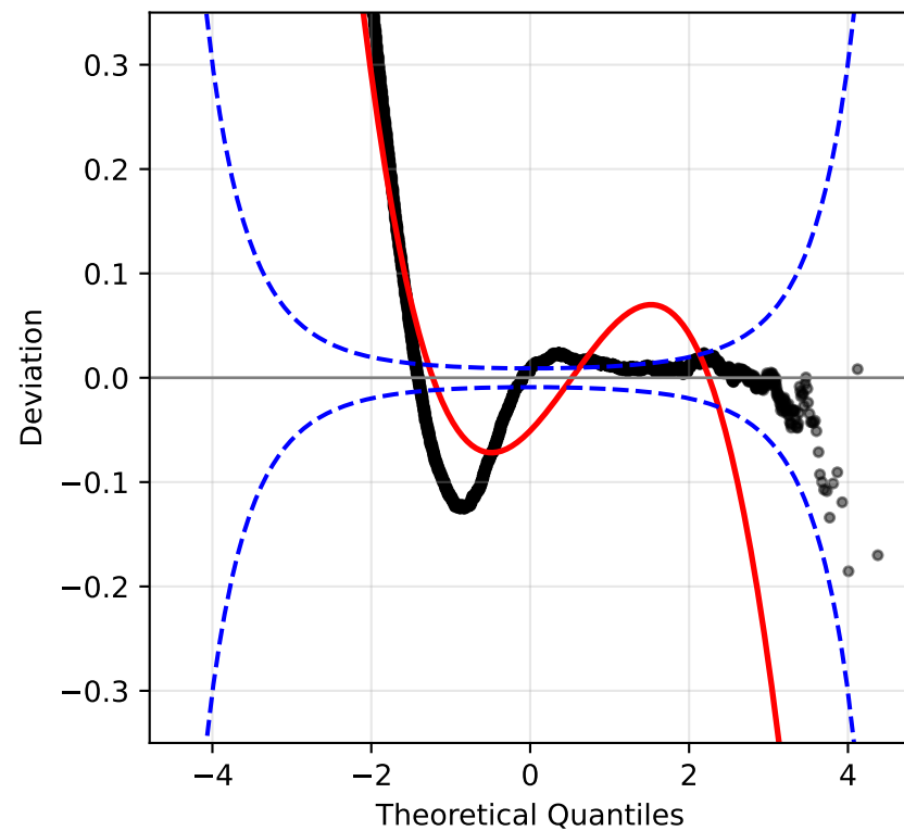
BS
