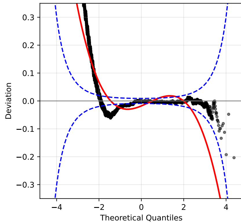
BS
