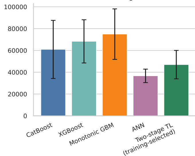
(d) RMSE \geq \text{training Q3} (USD)
