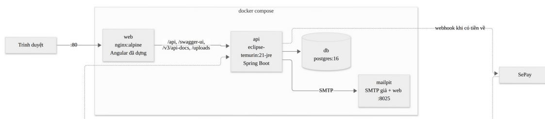
Hình 2.1 — Kiến trúc tổng thể của hệ thống khi triển khai (Nguồn: tác giả)
