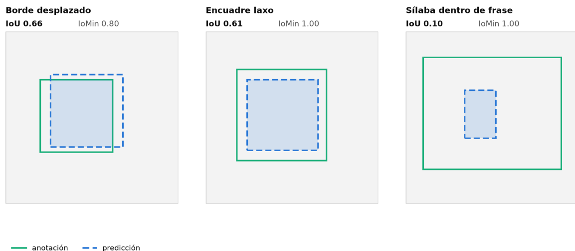
Figura 1.6: Criterio de IoU.
