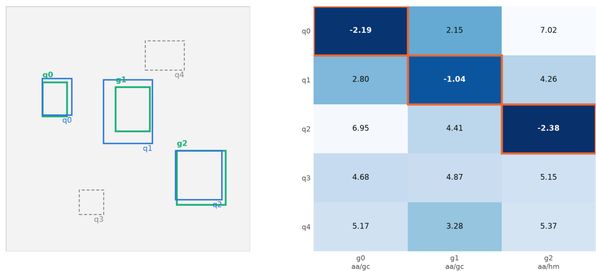
Figura 5.6: Emparejamiento húngaro.
