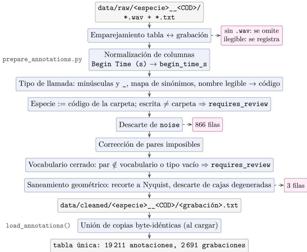
Figura 4.8: Reglas del protocolo en orden de aplicación
