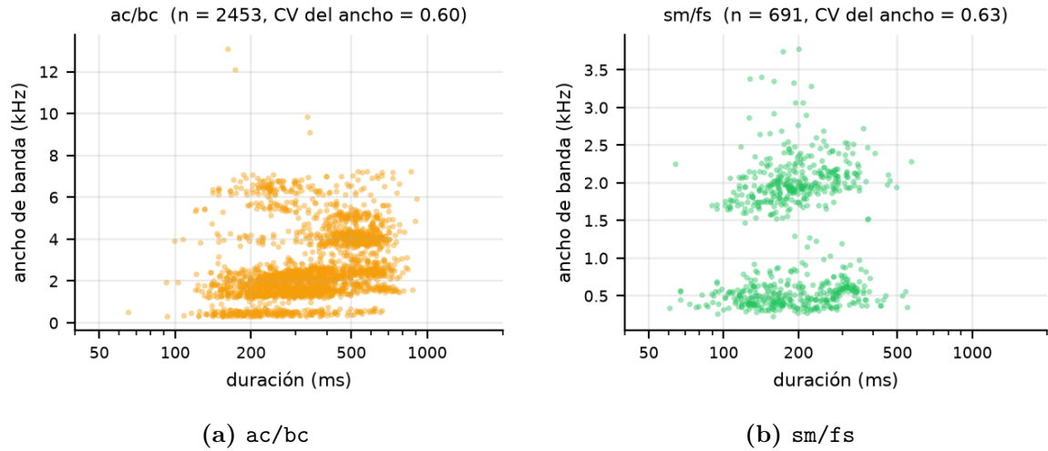
Figura 4.21: Duración frente a ancho de banda: dos nubes bajo una misma etiqueta
