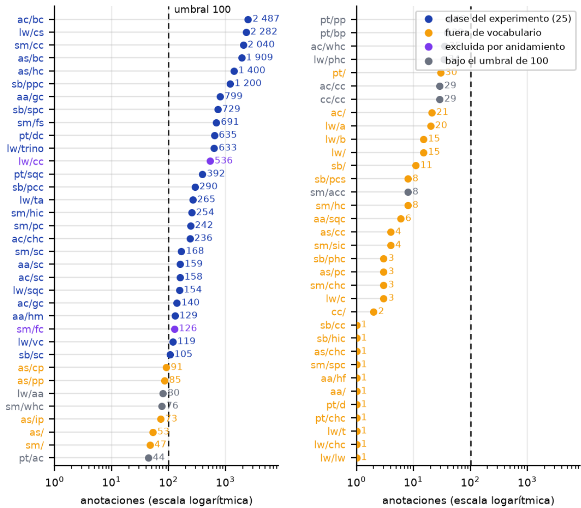
Figura 4.10: Anotaciones por par de especie y tipo de llamada en data/cleaned/ , con el umbral del experimento. La cola larga llega hasta pares con una sola anotación.
