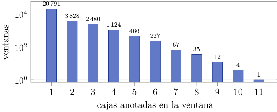
Figura 4.15: Cajas anotadas por ventana, sobre las ventanas con al menos una (escala logarítmica)
