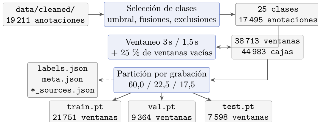
Figura 4.9: De las anotaciones curadas al caché de ventanas ( src/prepare_data.py )
