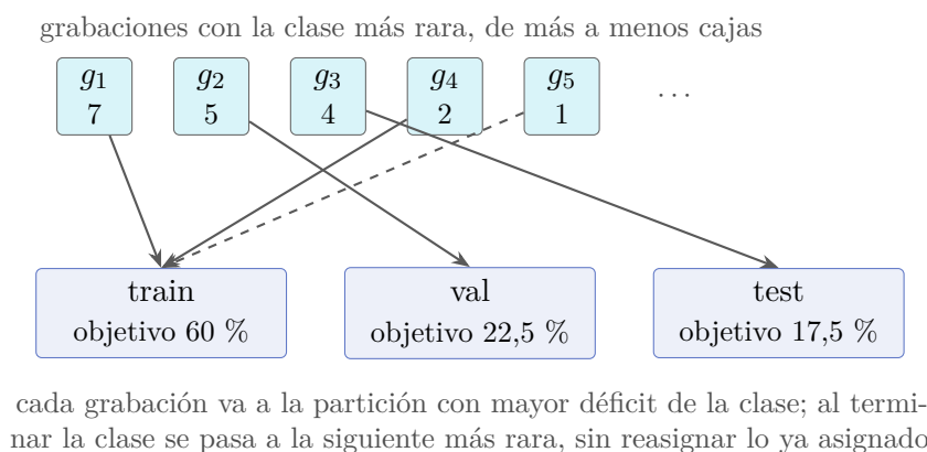
Figura 4.12: Reparto goloso por grabación, estratificado por clase (bajo cada grabación, sus cajas de la clase en reparto)
