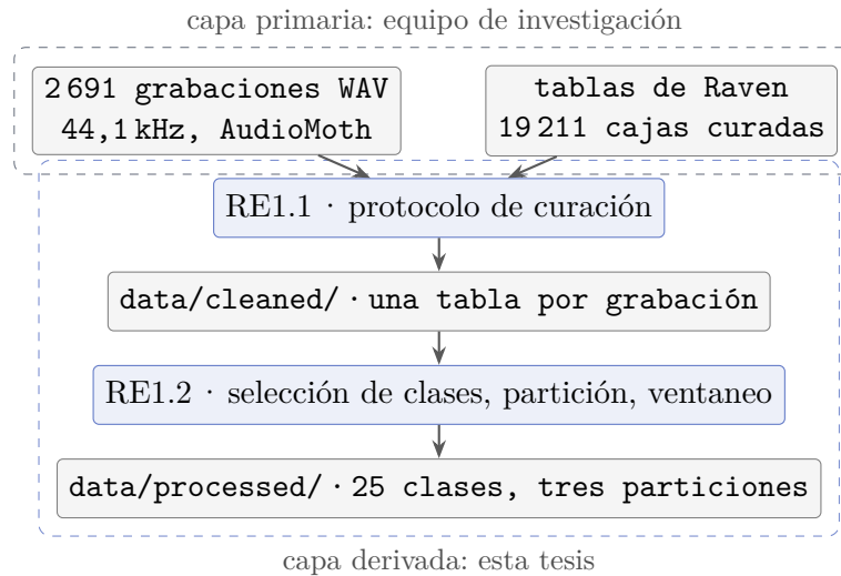
Figura 4.18: Capas del conjunto y responsable de cada una
