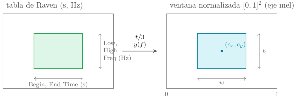
Figura 4.16: Normalización de una caja: el tiempo por la longitud de la ventana, la frecuencia por la escala mel
