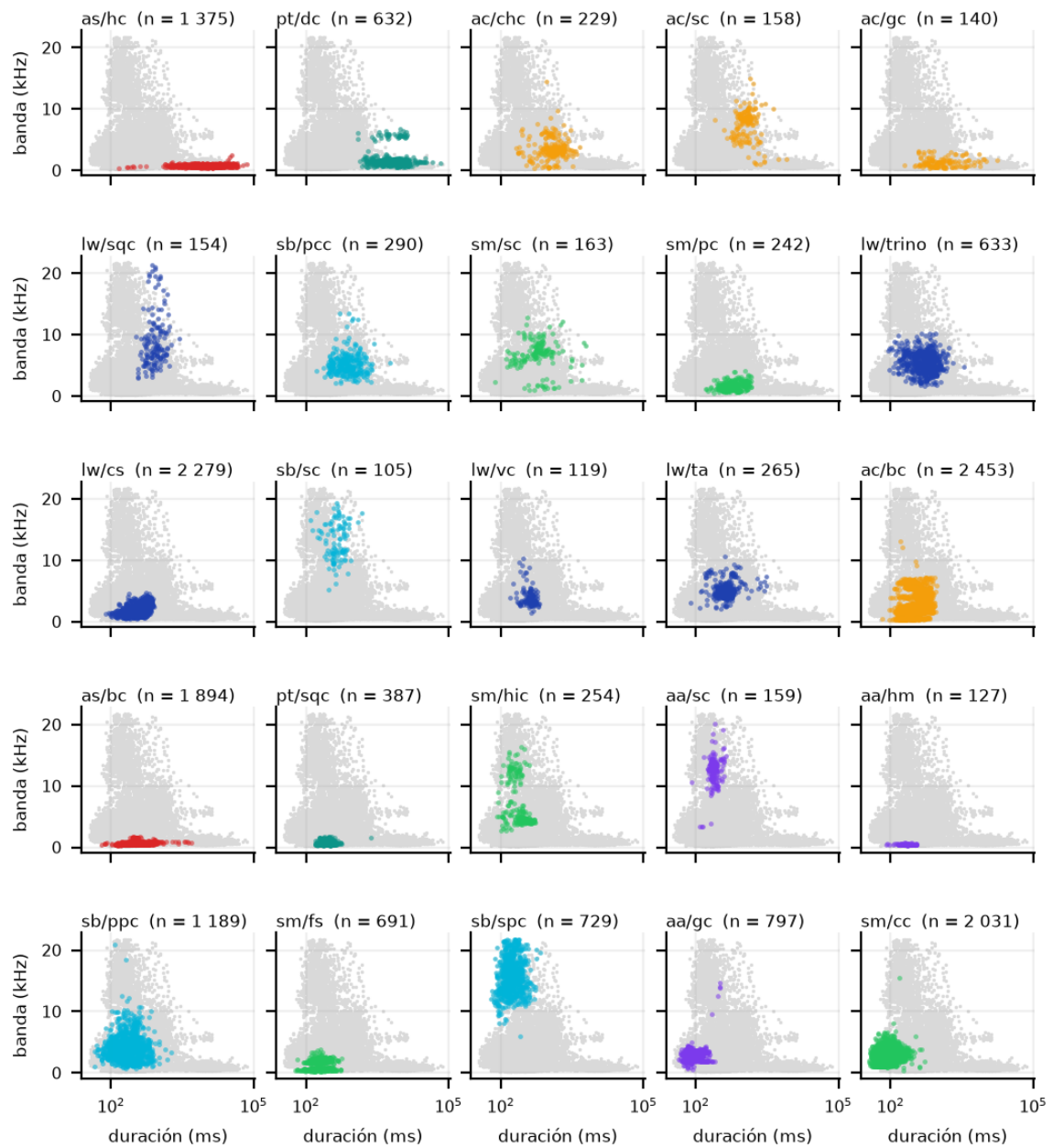
Figura 4.20: Duración frente a ancho de banda, un panel por clase del experimento. En gris, todas las clases; en color, la del panel.
