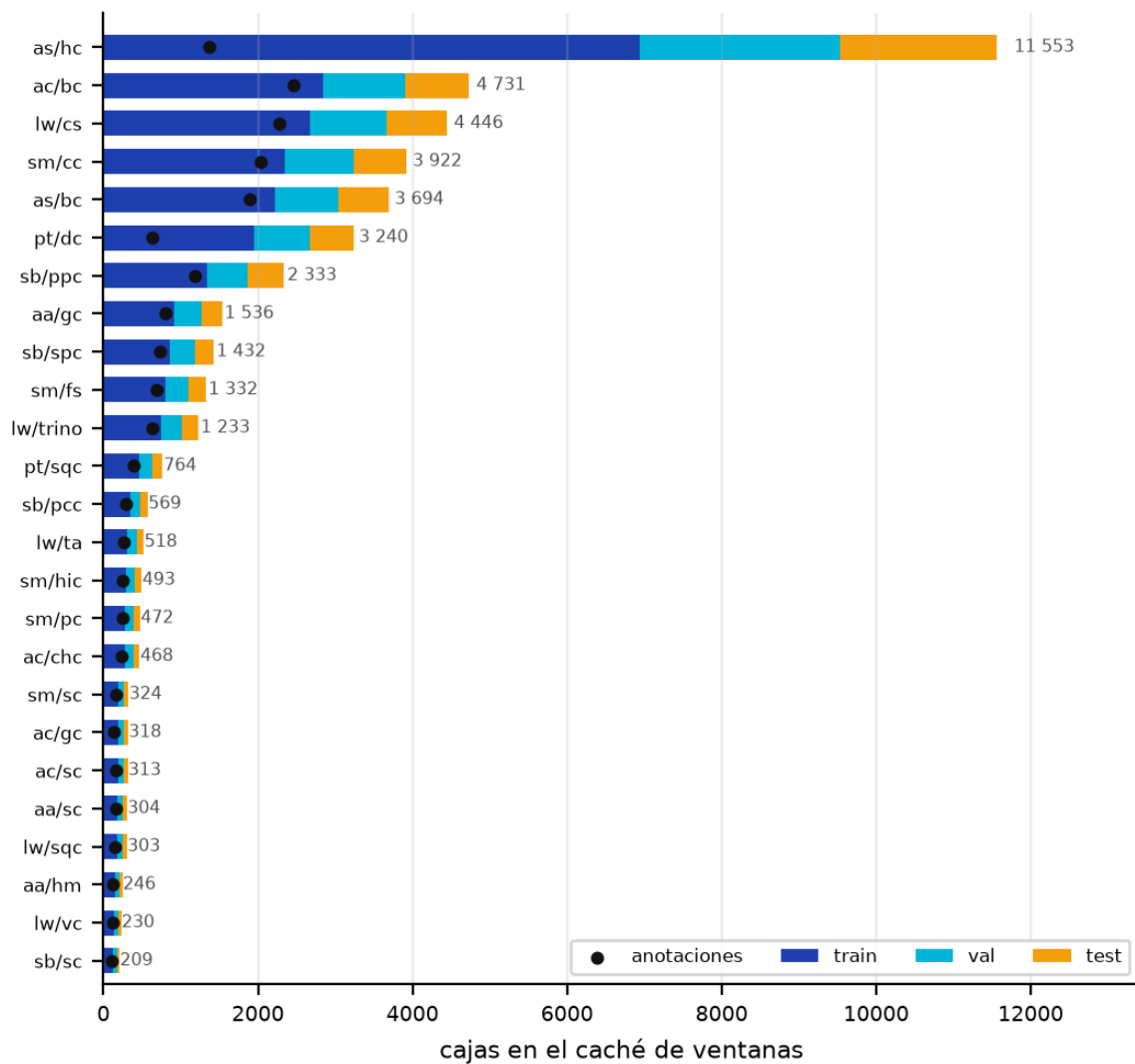
Figura 4.13: Cajas por clase y partición, con las anotaciones de la clase como referencia. La proporción entre particiones se conserva; el desbalance entre clases se mantiene, y la distancia entre las cajas y las anotaciones es lo que el ventaneo multiplica.
