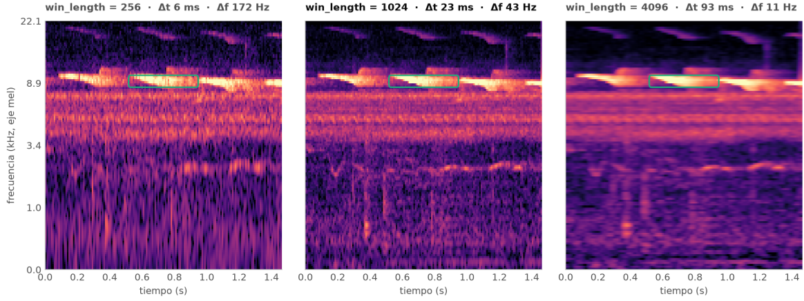
Figura 2.3: Compromiso STFT.
