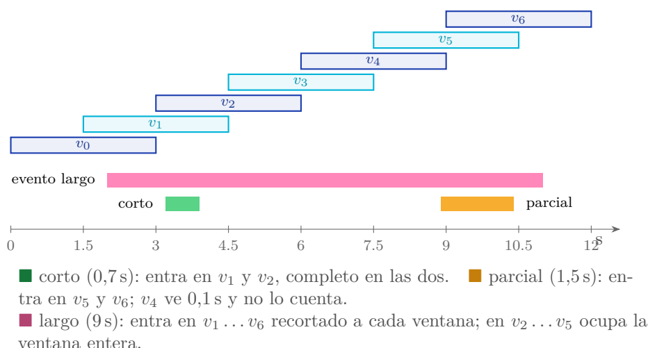
Figura 4.14: Asignación de eventos a ventanas de 3 s con salto de 1,5 s
