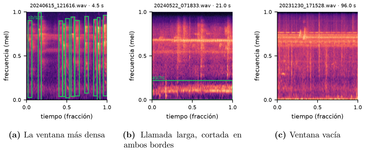
Figura 4.17: Ventanas de entrenamiento tal como las recibe el modelo (mel en dB, cajas normalizadas)
