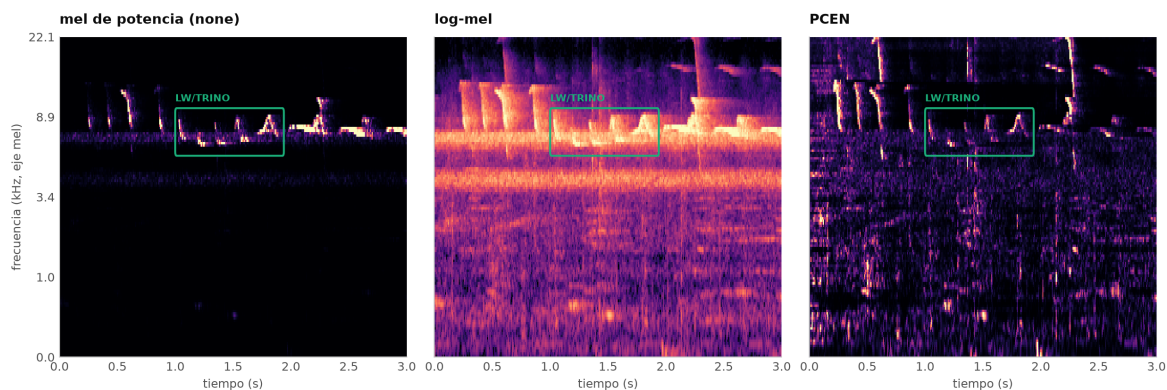
Figura 2.5: Los tres front-ends de entrada del detector sobre la misma ventana: mel de potencia sin transformar, log-mel y PCEN.
