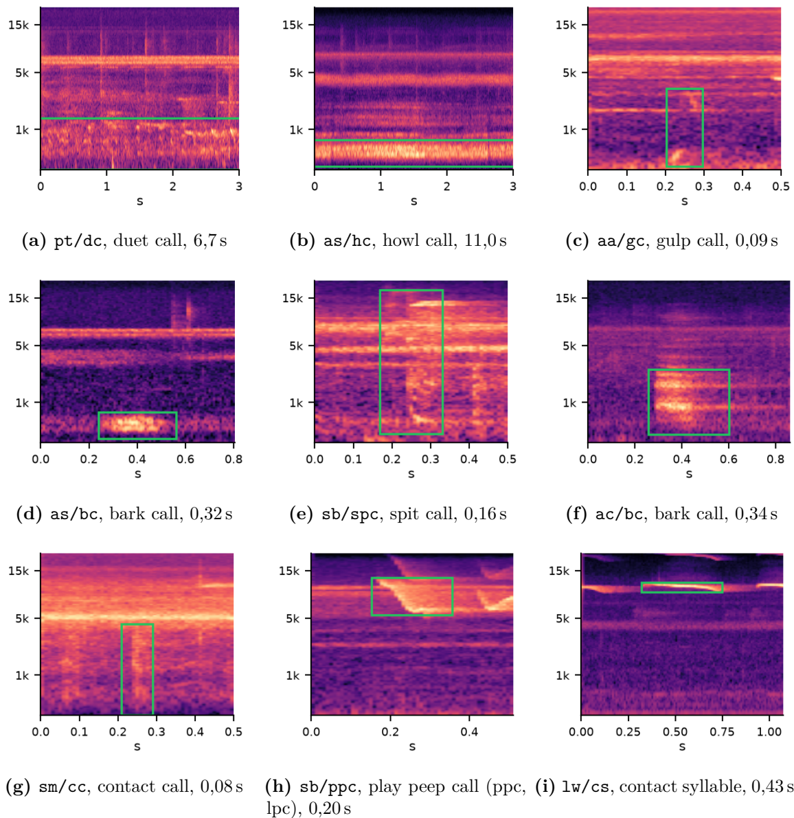
Figura 4.19: 9 clases sobre el espectrograma (anotación en verde; eje de frecuencia en escala mel). De cada clase, la anotación de duración más cercana a la mediana de su clase; en las dos clases largas el evento excede el panel de 3 s y la caja se sale por los lados.
