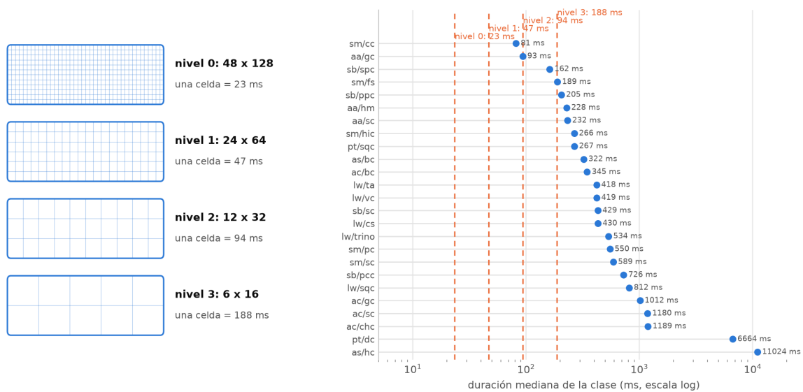
Figura 5.2: Pirámide multiescala.
