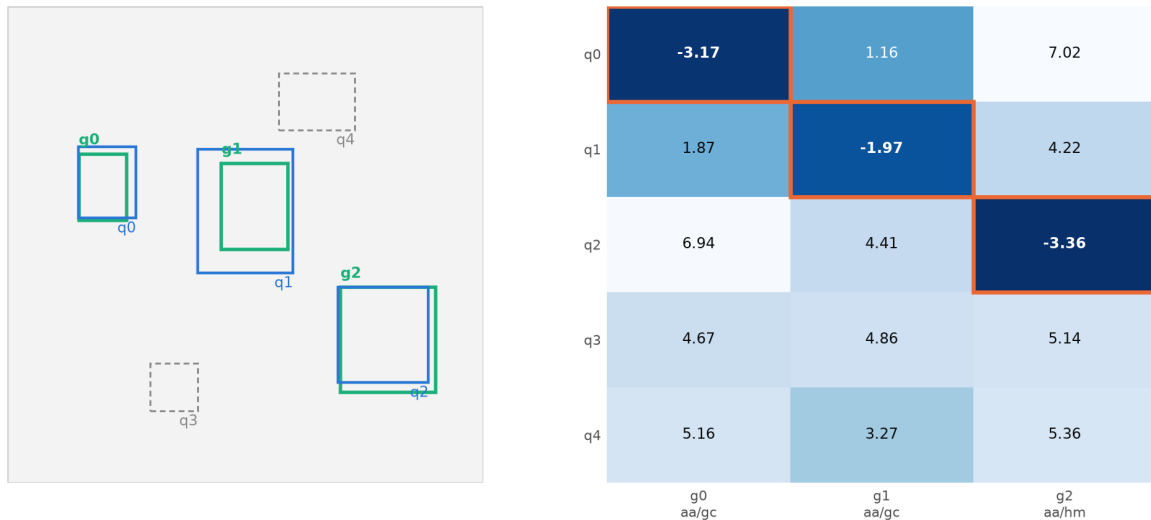
Figura 5.6: Emparejamiento húngaro.
