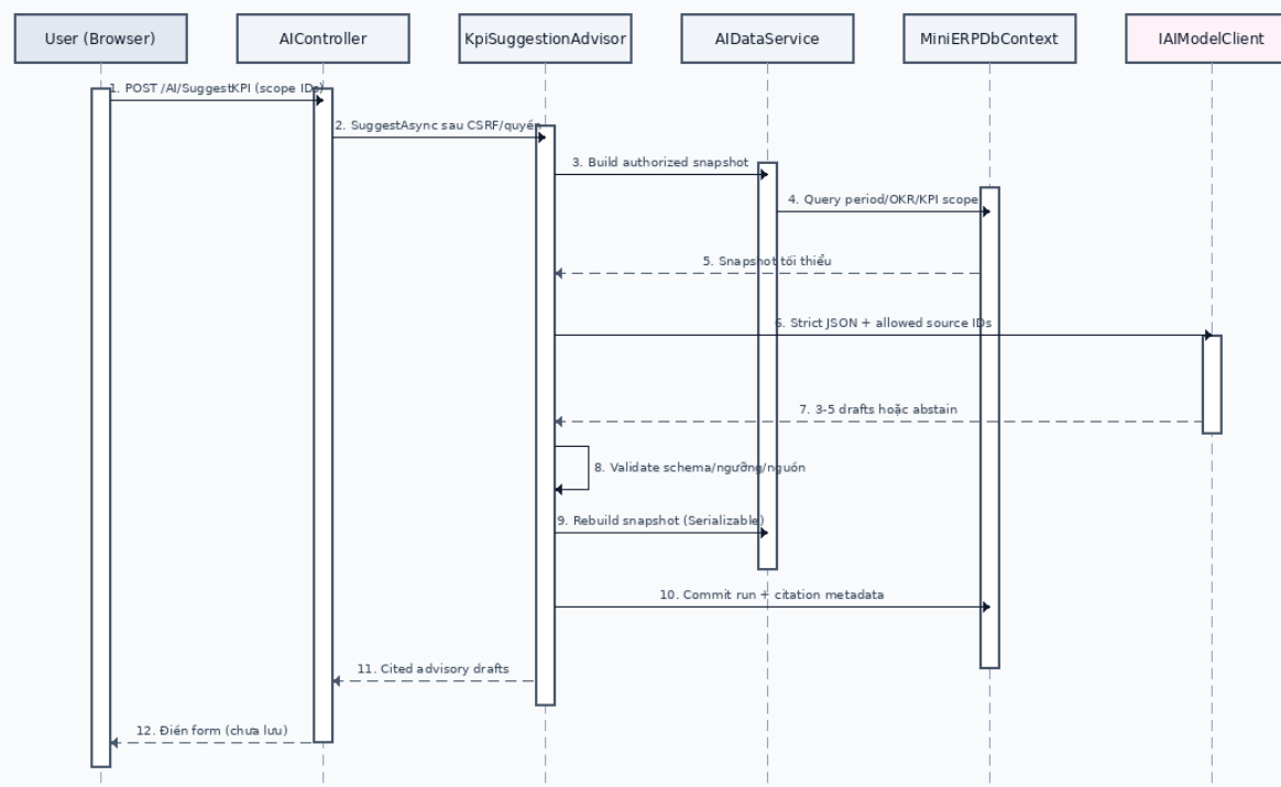
SƠ ĐỒ TUẦN TỰ: KPI SUGGESTION ADVISOR CÓ NGUỒN
