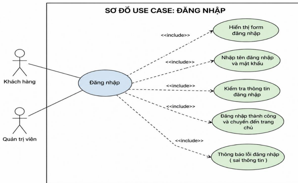
Hình 2-5: Sơ đồ use case đăng nhập
