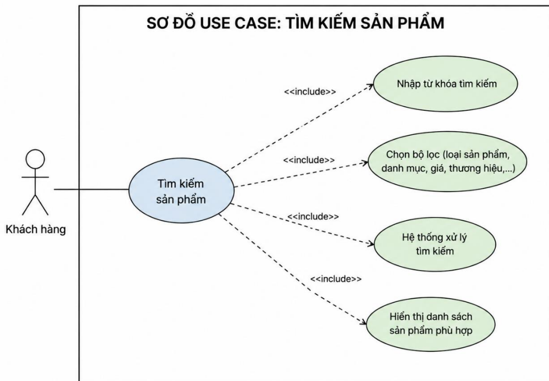
Hình 2-7: Sơ đồ use case Tìm kiếm sản phẩm
