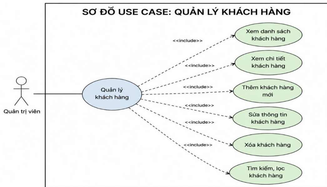
Hình 2-13: Sơ đồ use case Quản lý khách hàng
