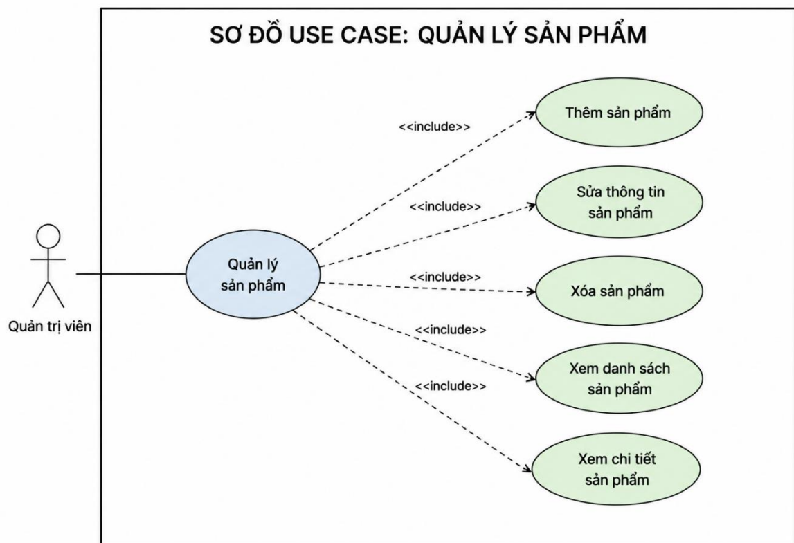
Hình 2-10: Sơ đồ use case Quản lý sản phẩm
