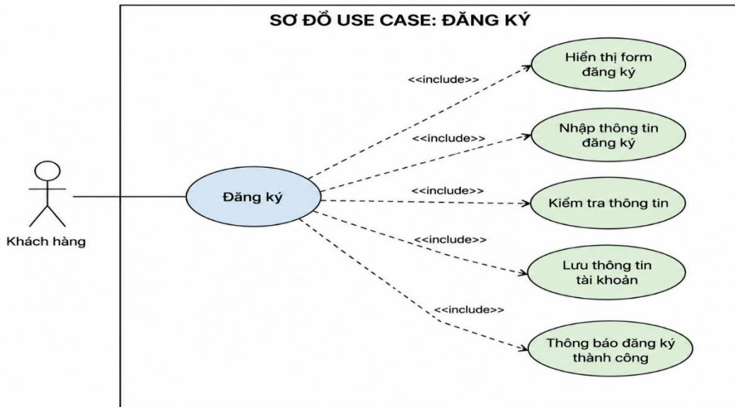
Hình 2-4: Sơ đồ use case đăng ký
