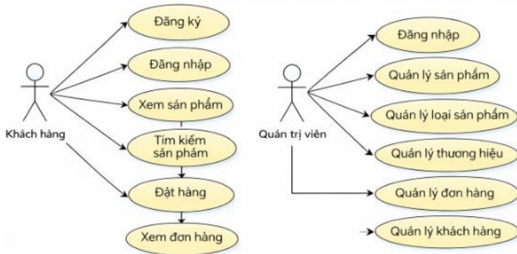
Hình 2-3: Sơ đồ Use Case hệ thống
