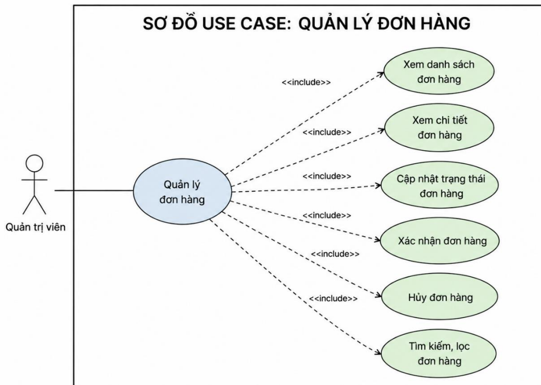
Hình 2-12: Sơ đồ use case quản lý đơn hàng
