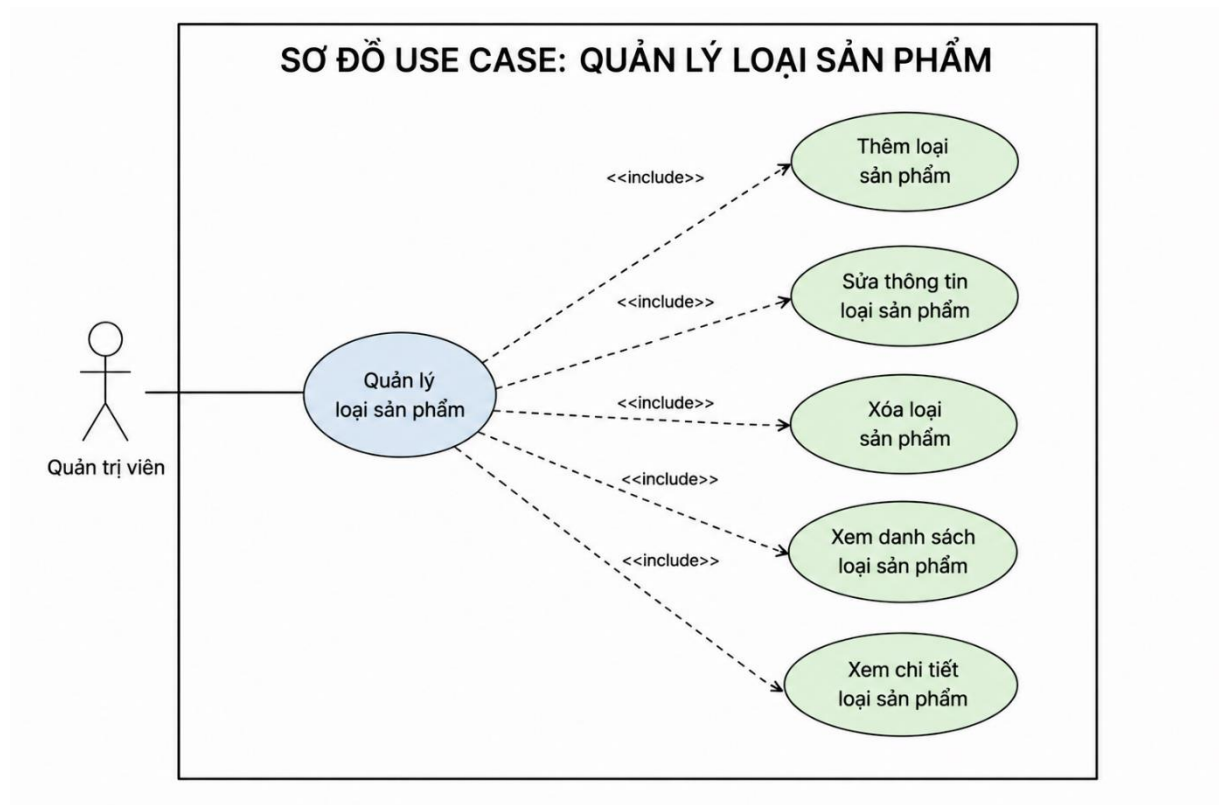
Hình 2-11: Sơ đồ use case quản lý loại sản phẩm
