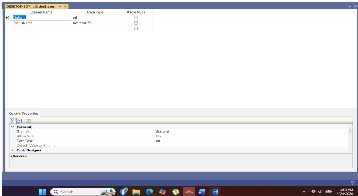
Hình 2-27: Bảng OrderStatus
