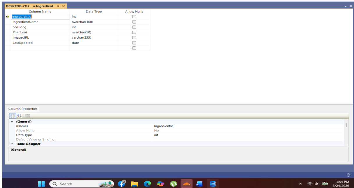
Hình 2-28: Bảng Ingredient
