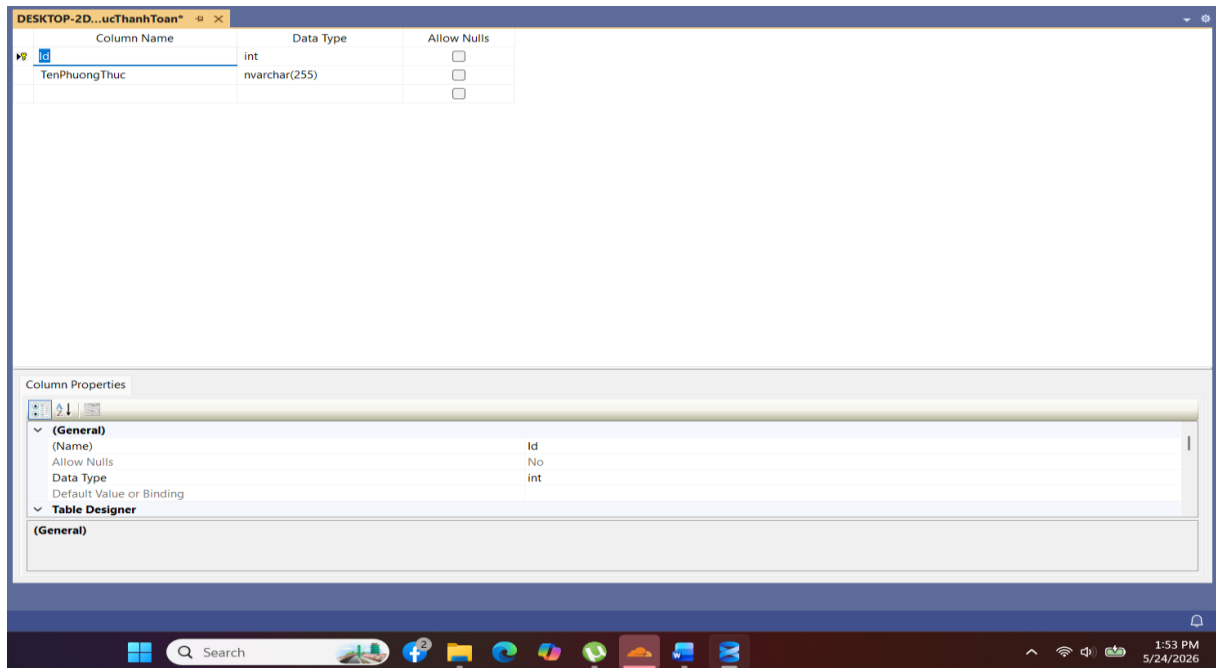
Hình 2-26: Bảng PhươngThucThanhToan
