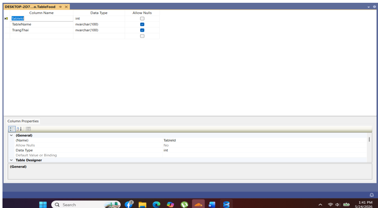
Hình 2-17: Bảng TableFood
