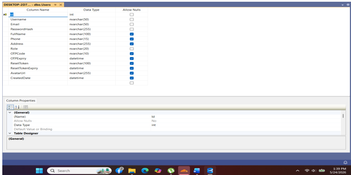
Hình 2-16: Bảng Users
