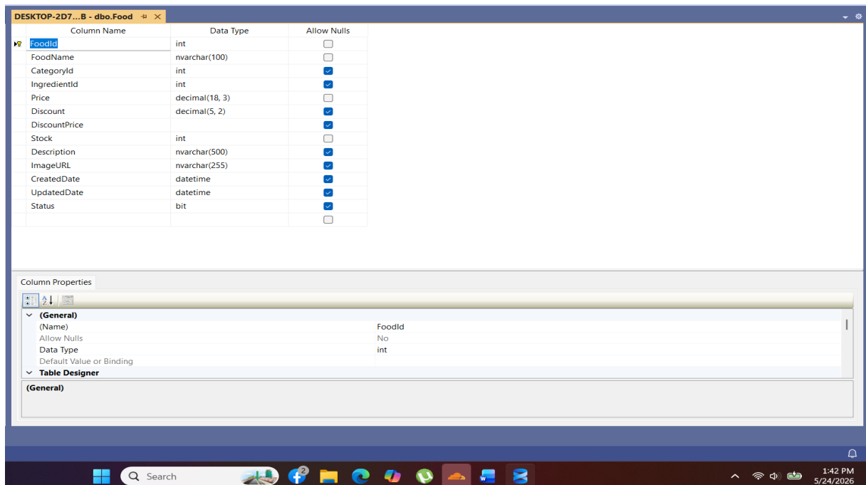
Hình 2-19: Bảng Food
