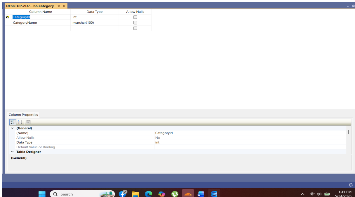
Hình 2-18: Bảng Category
