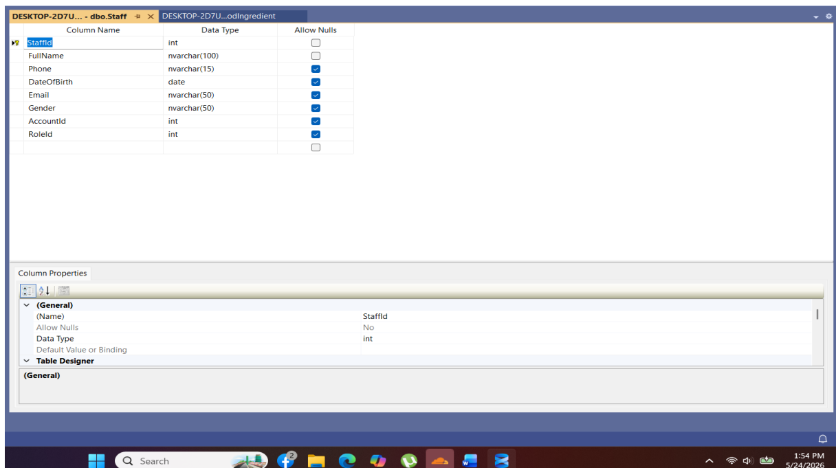
Hình 2-29: Bảng Staff
