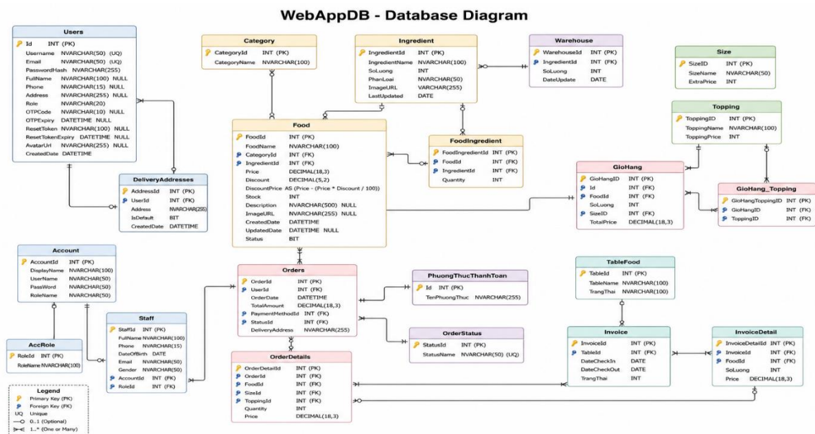
Hình 2-2: Sơ đồ cơ sở dữ liệu (Database Diagram)
