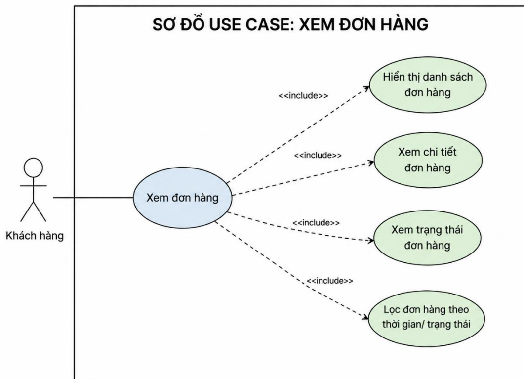
Hình 2-9: Sơ đồ use case Xem đơn hàng
