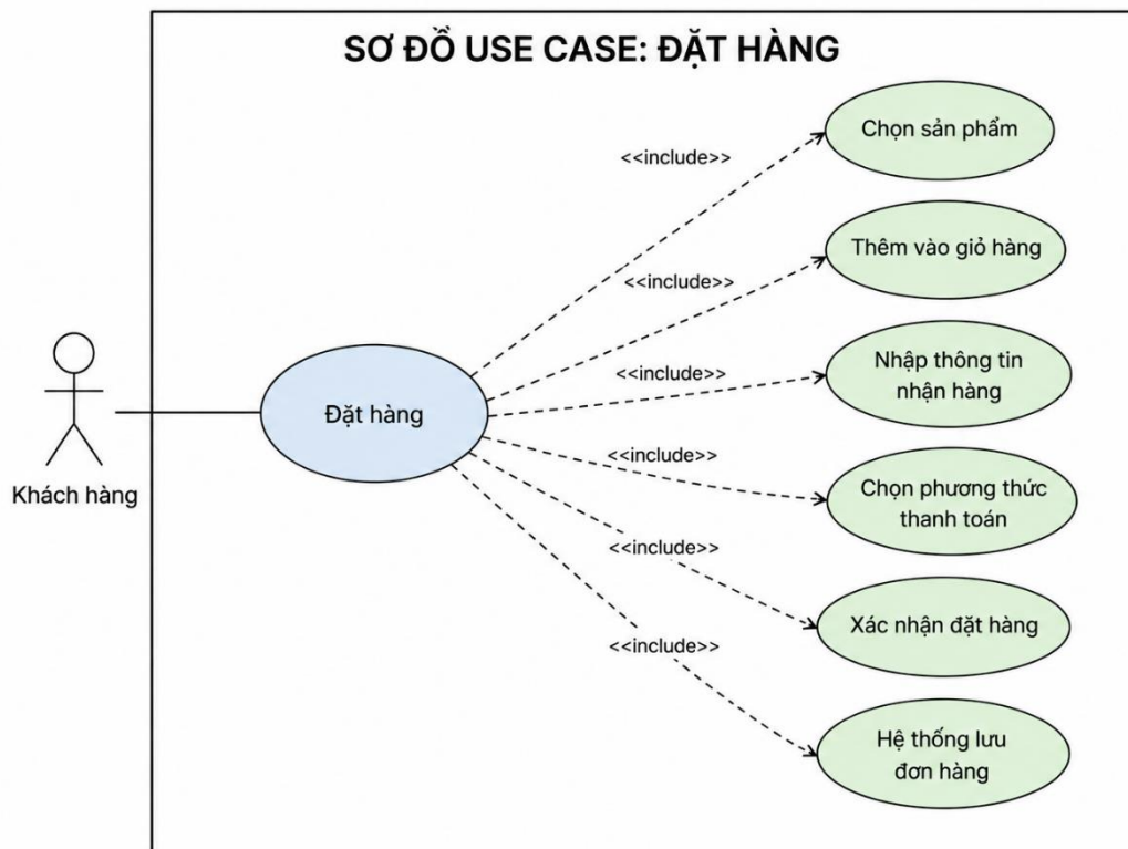
Hình 2-8: Sơ đồ use case Đặt hàng
