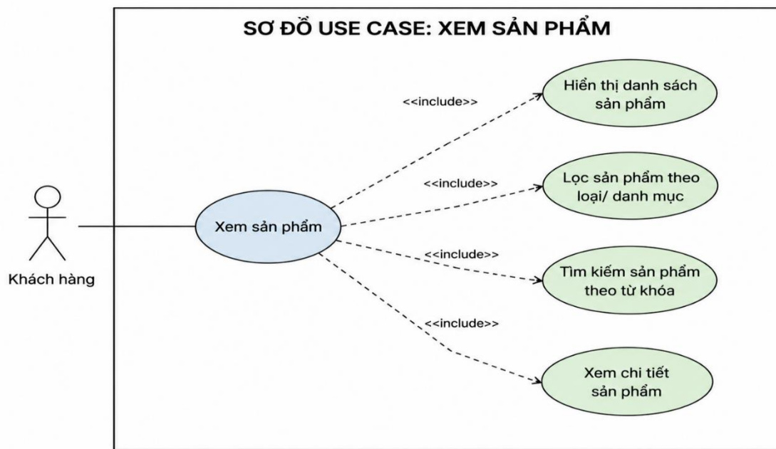
Hình 2-6: Sơ đồ use case xem sản phẩm
