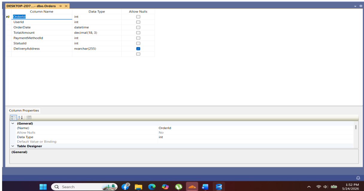
Hình 2-24: Bảng Orders
