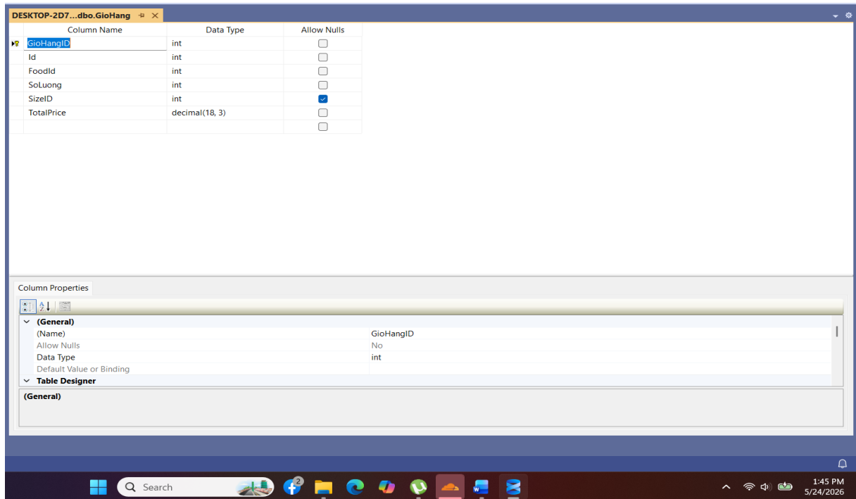
Hình 2-22: Bảng GioHang
