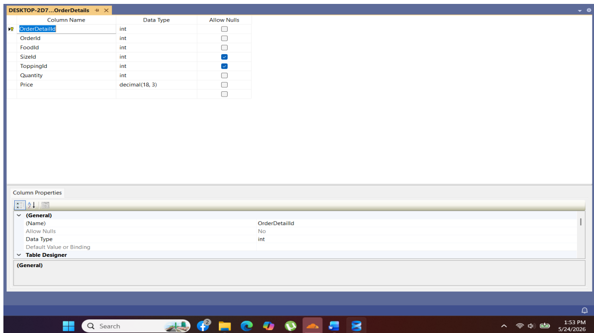
Hình 2-25: Bảng OrderDetails
