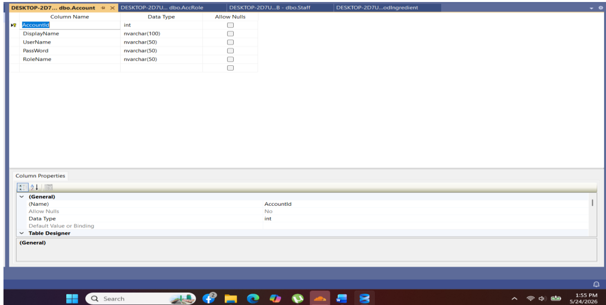
Hình 2-30: Bảng Account
