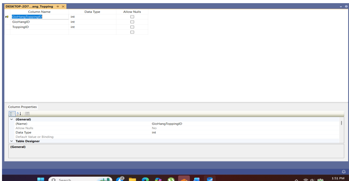
Hình 2-23: Bảng GioHang_Topping
