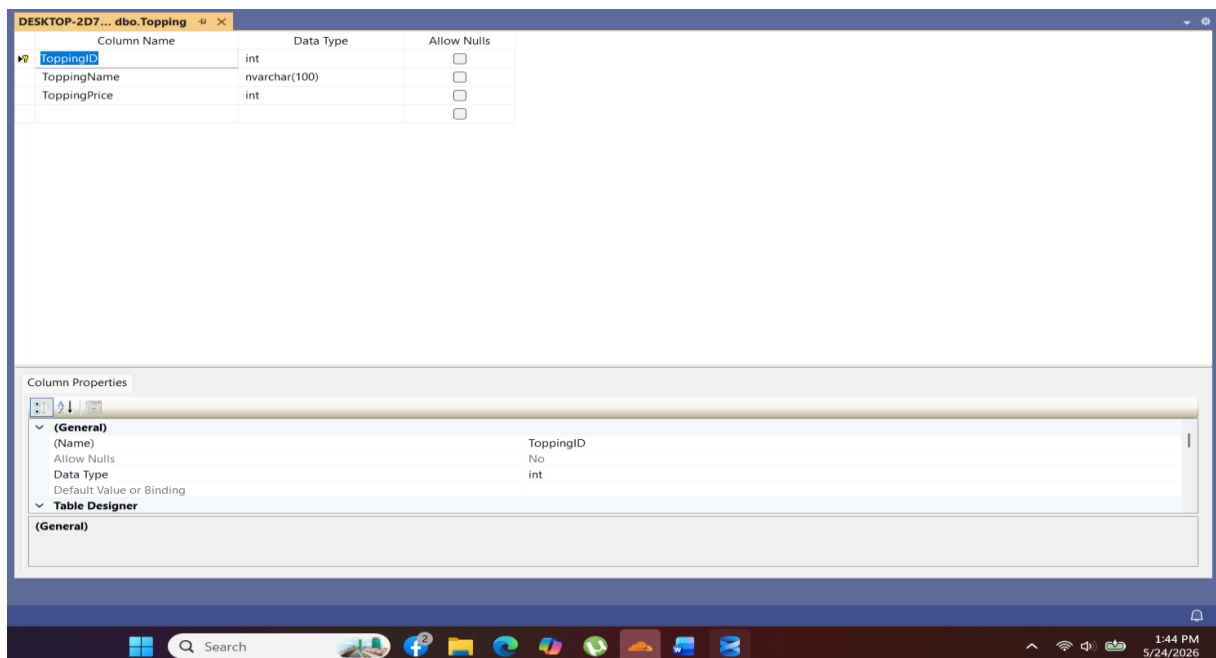
Hình 2-21: Bảng Topping
