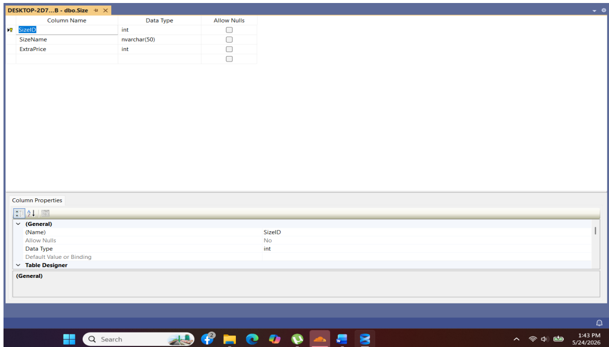
Hình 2-20: Bảng Size
