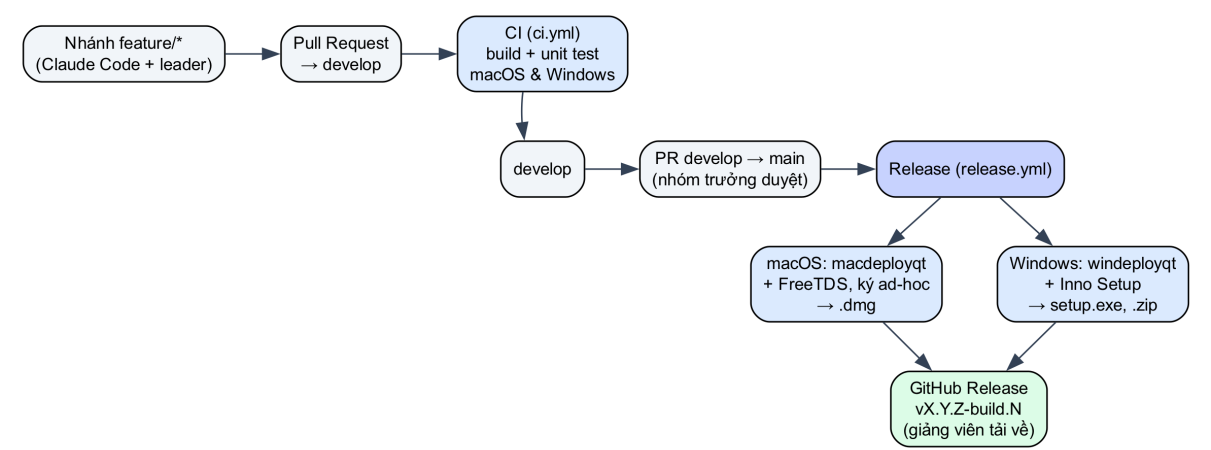
Hình 6.9. Quy trình CI/CD từ nhánh tính năng tới file cài
