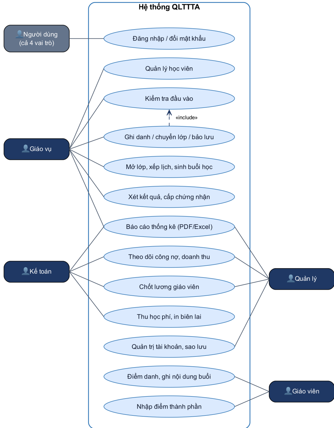
Hình 2.1. Sơ đồ use case tổng quát của hệ thống QLTTTA
