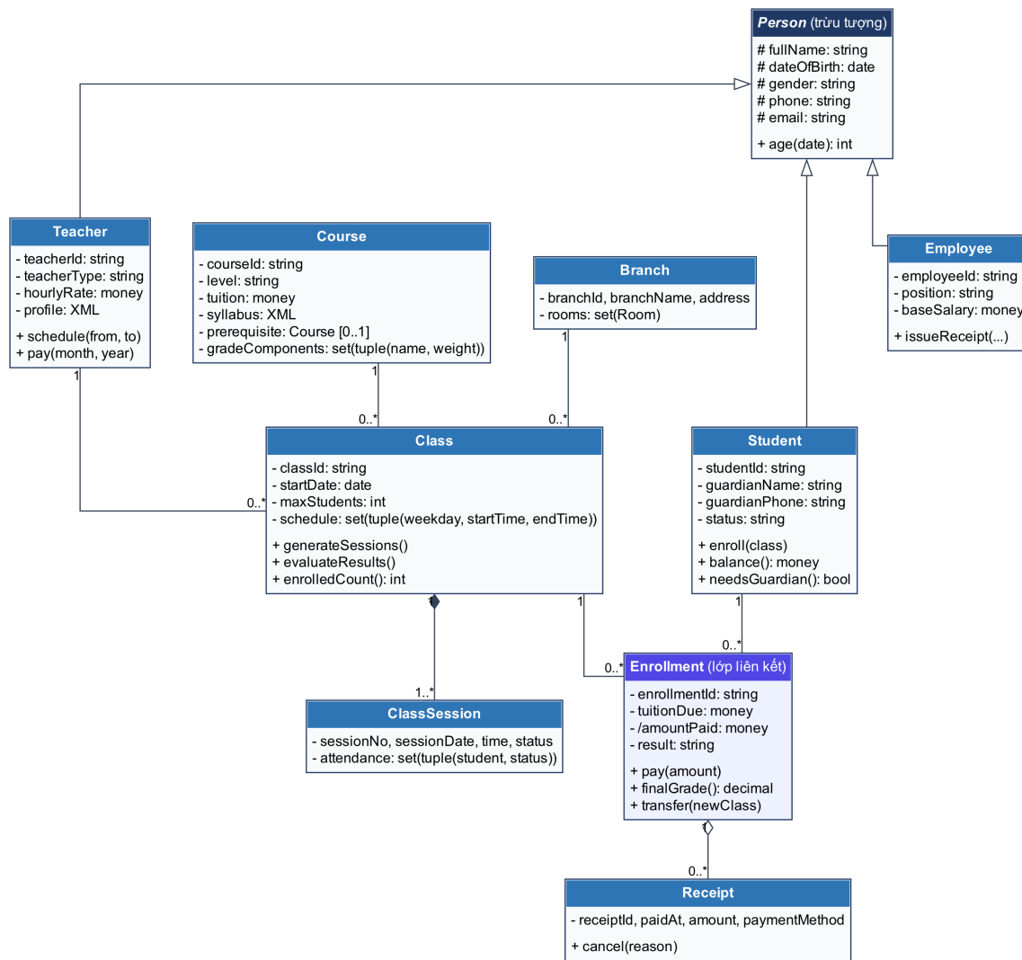
Hình 3.3. Sơ đồ lớp (CD) của hệ thống QLTTA
