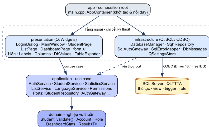
Hình 6.1. Clean Architecture của ứng dụng QLTTTA
