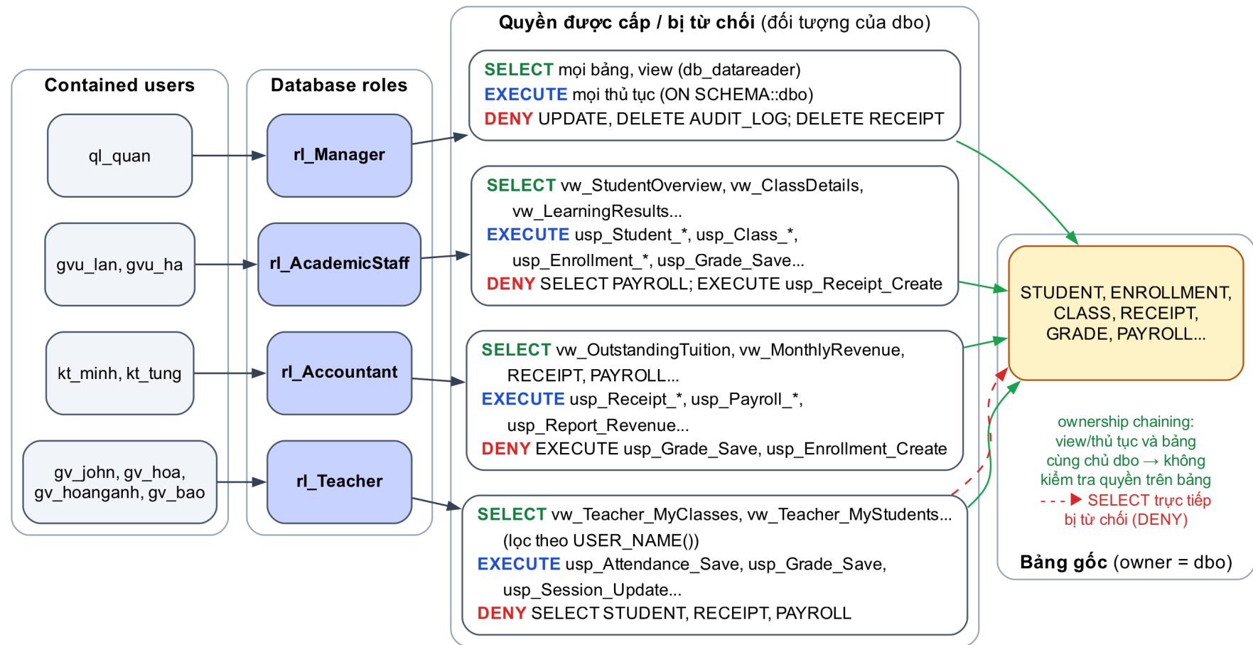
Hình 5.1. Phân quyền: user → role → view/thủ tục → bảng
